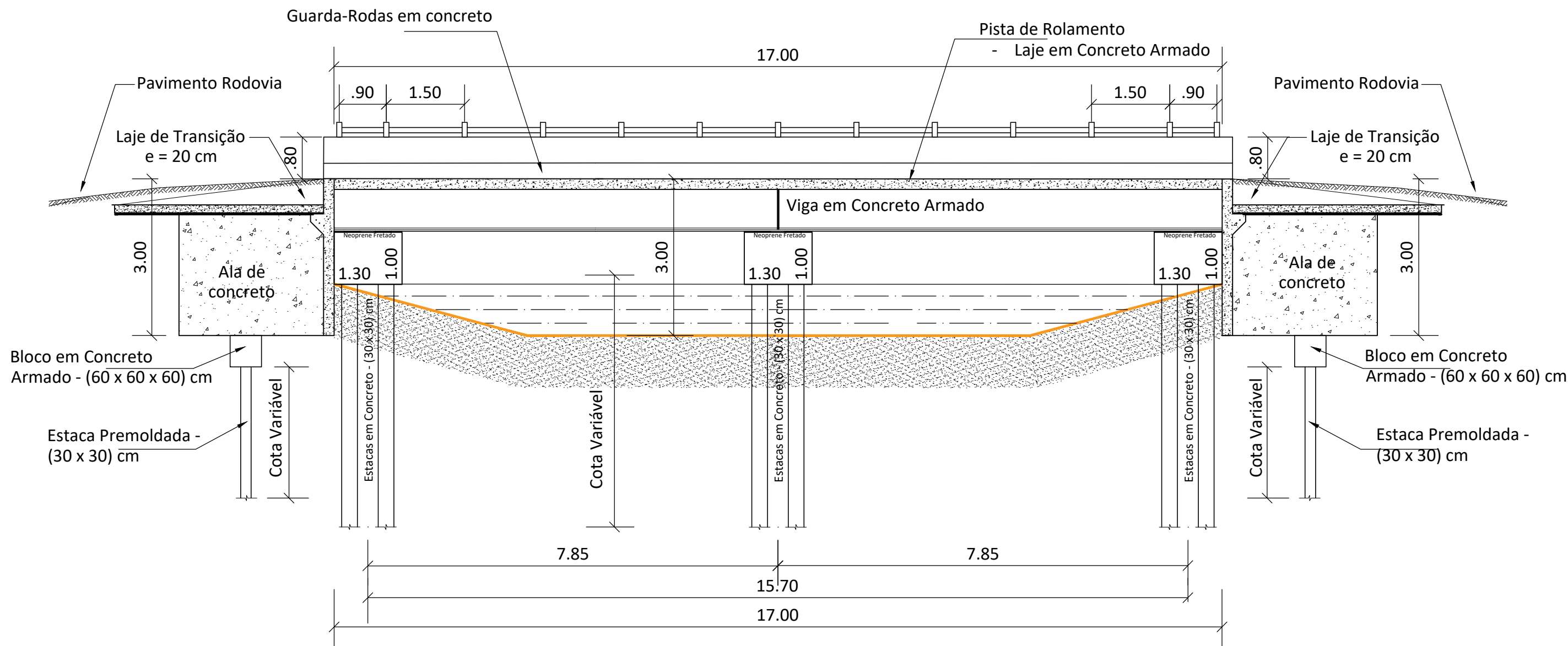
SEÇÃO 01 - LONGITUDINAL
