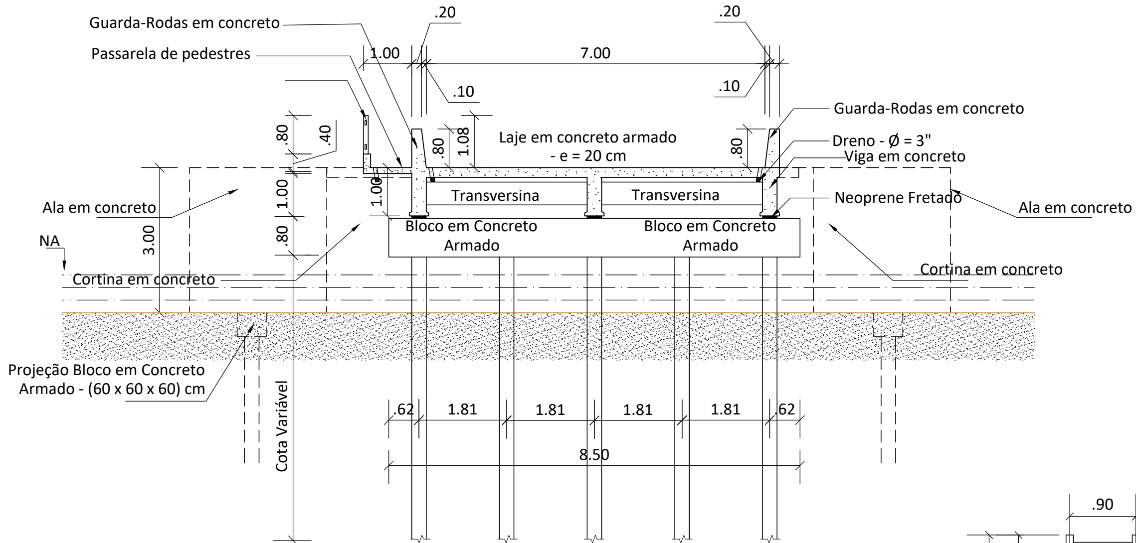
SEÇÃO 02 - TRANSVERSAL
