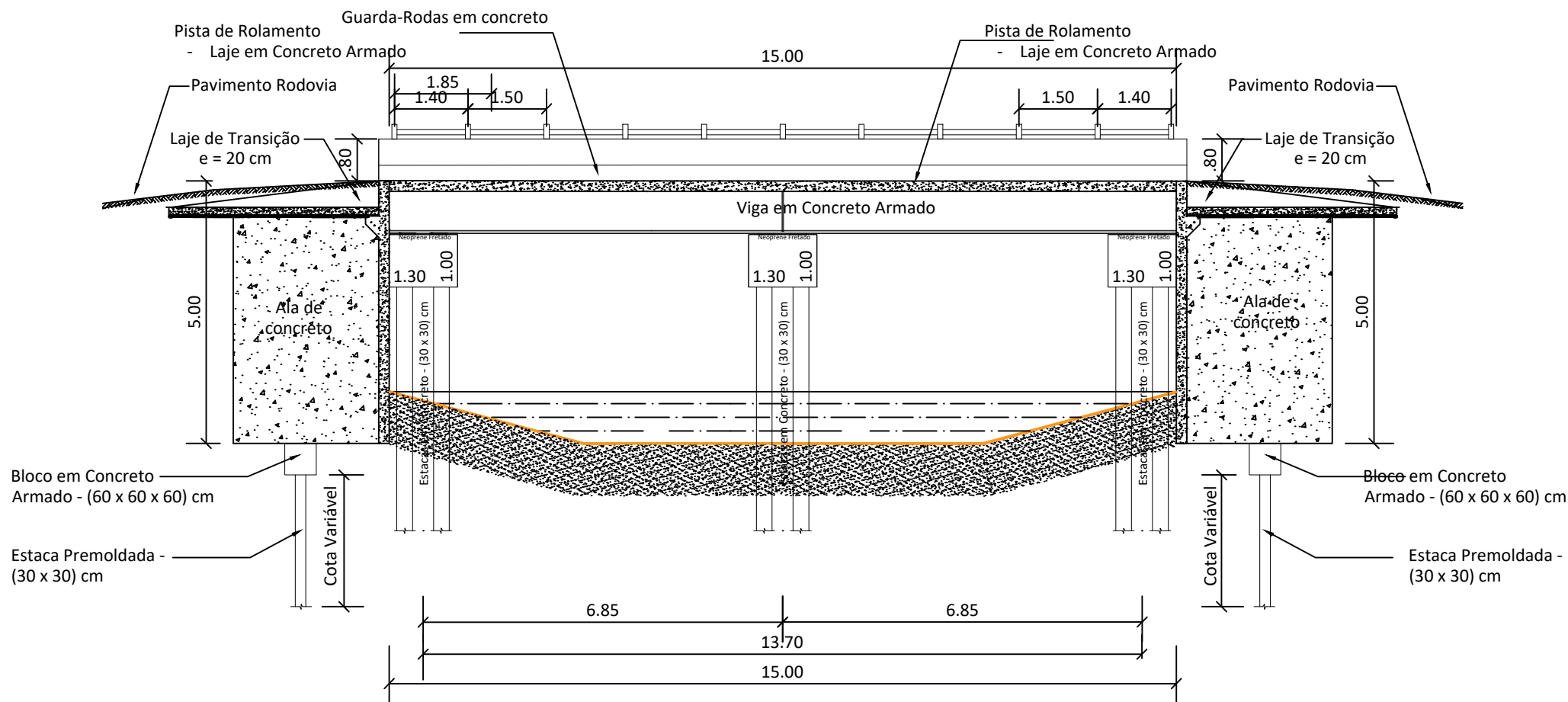
SEÇÃO 01 - LONGITUDINAL
