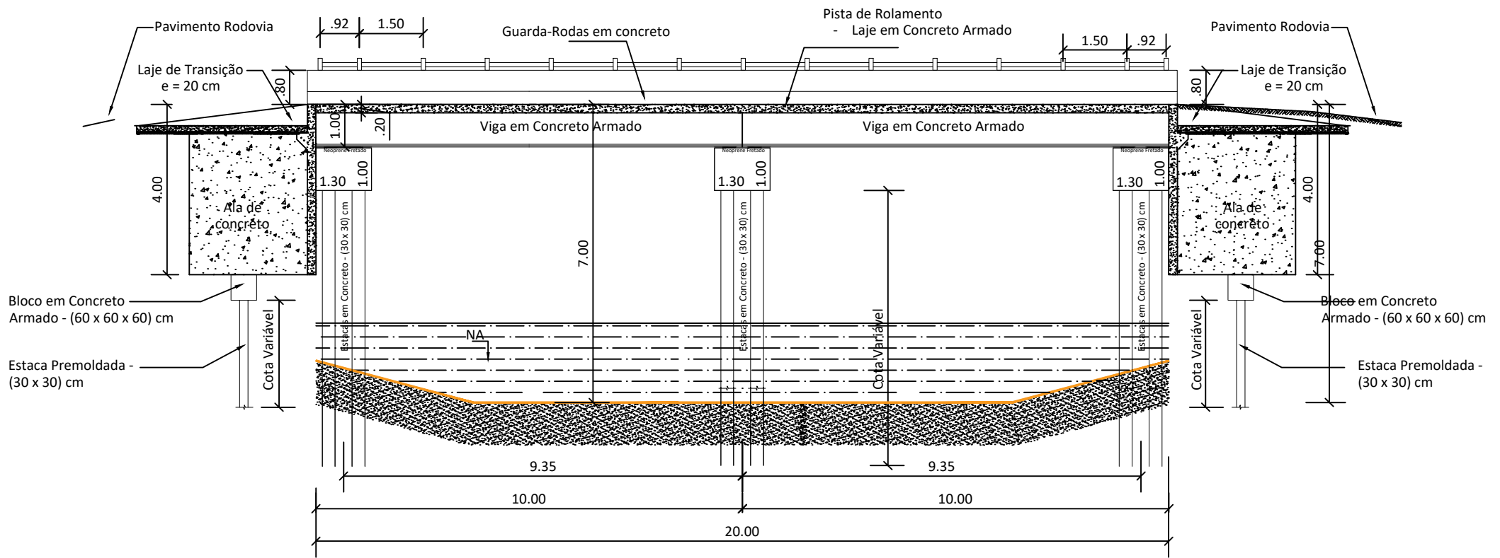
SEÇÃO 01 - LONGITUDINAL
