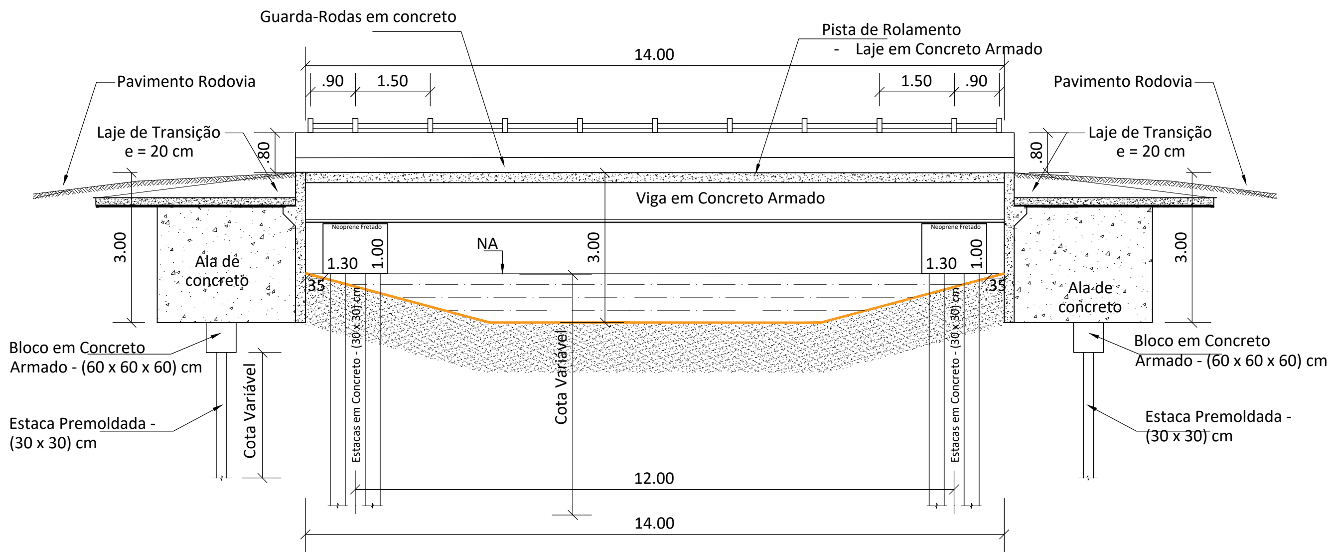
SEÇÃO 01 - LONGITUDINAL
