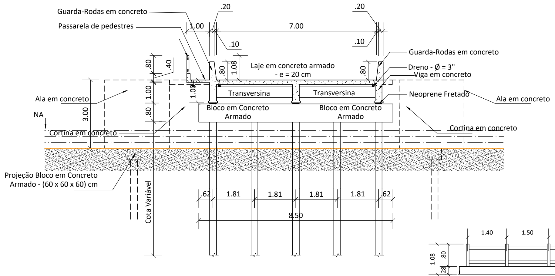
SEÇÃO 02 - TRANSVERSAL
