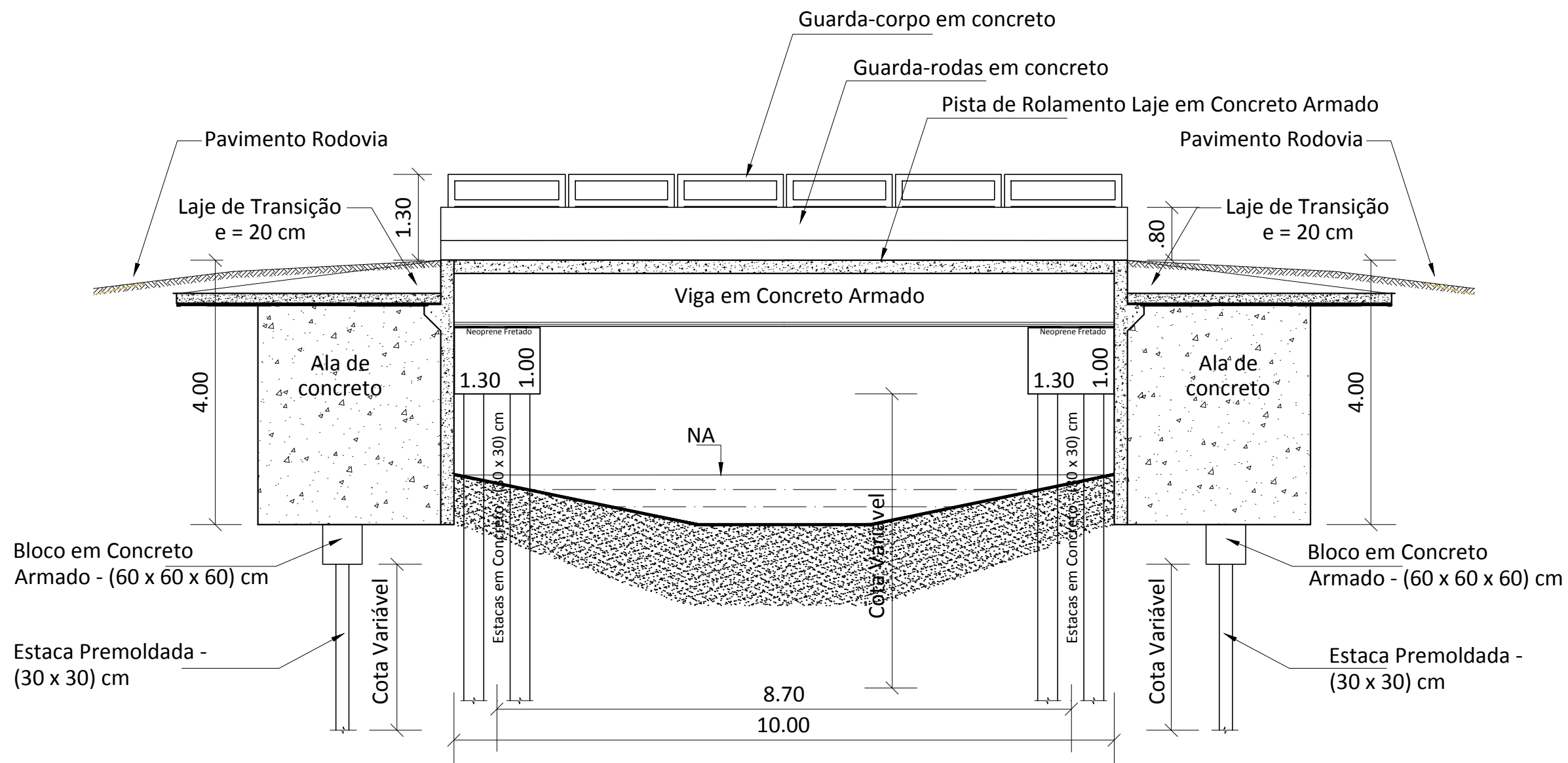
SEÇÃO 01 - LONGITUDINAL Escala: 1/75
