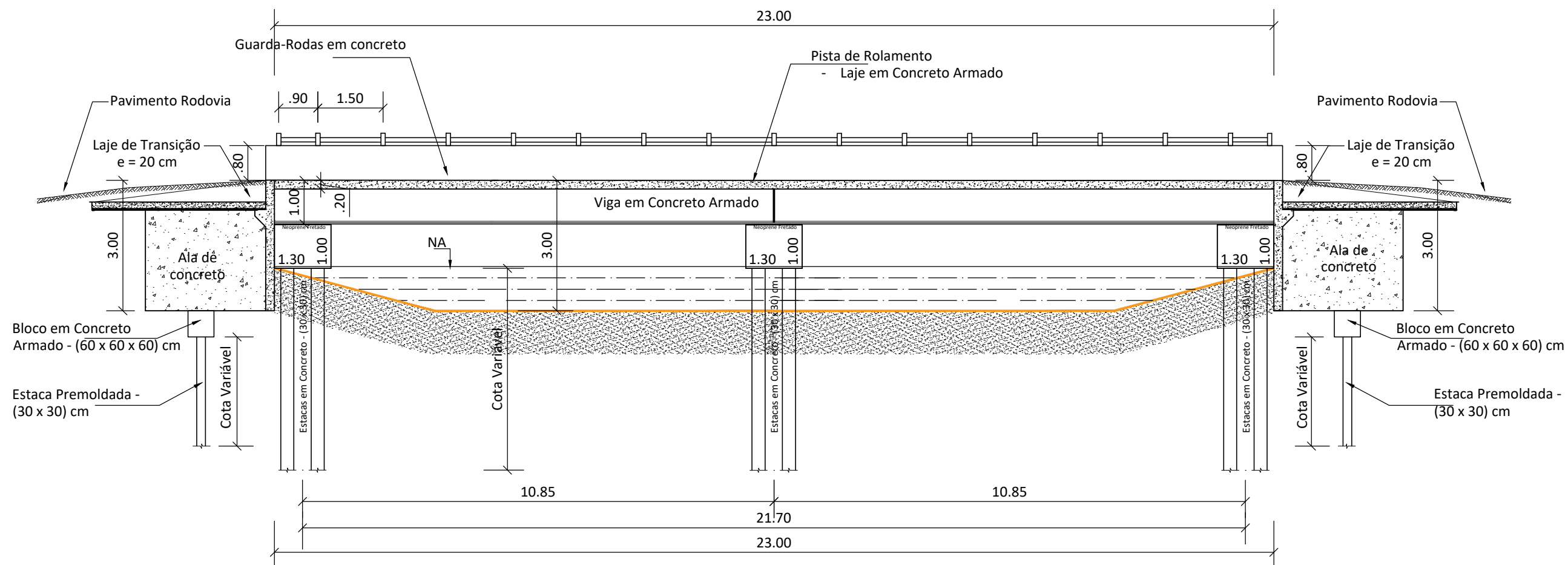
SEÇÃO 01 - LONGITUDINAL
