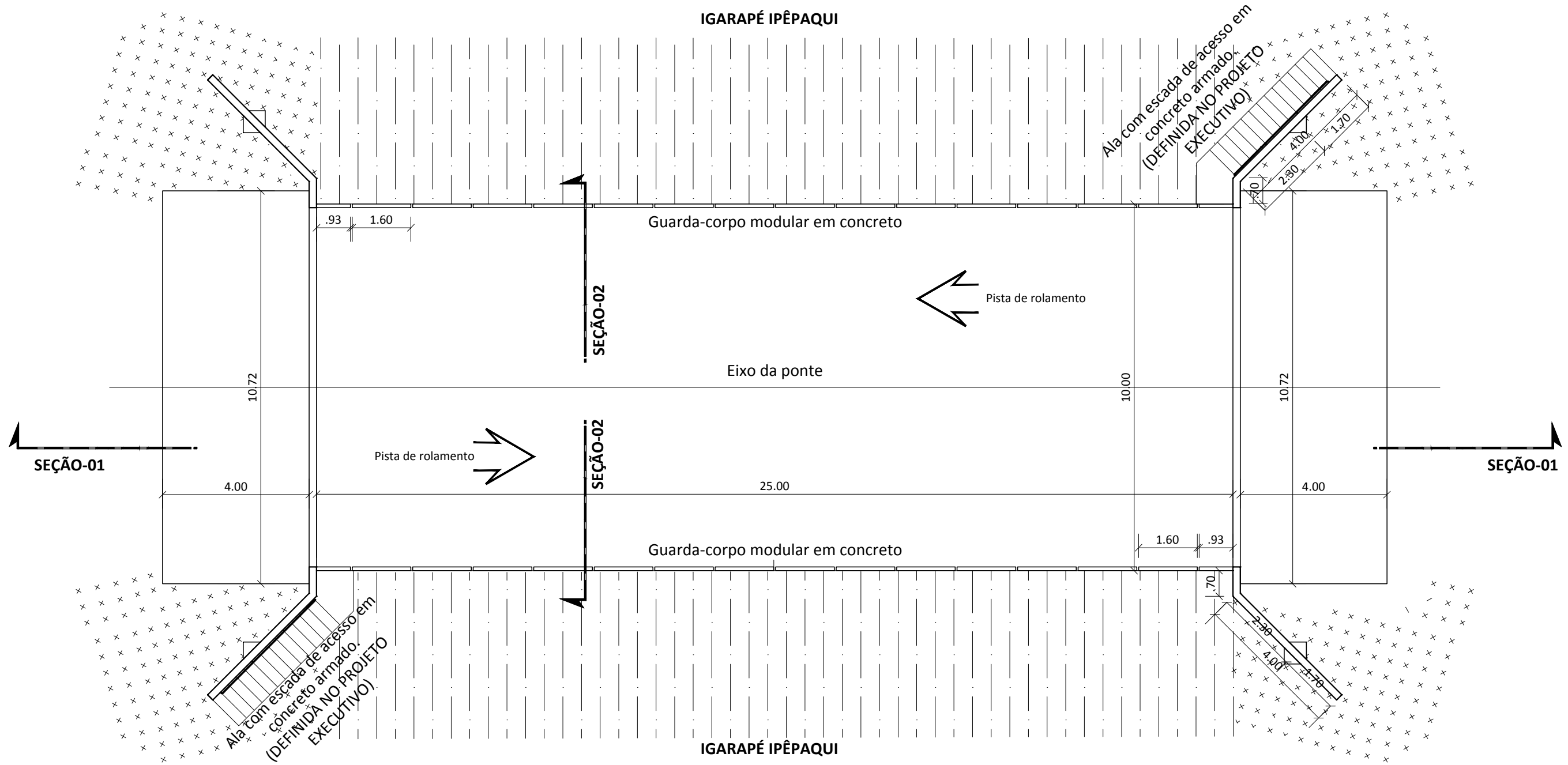
PLANTA ESQUEMÁTICA DA PONTE - IGARAPÉ IPÊPAQUI Escala: 1/125
