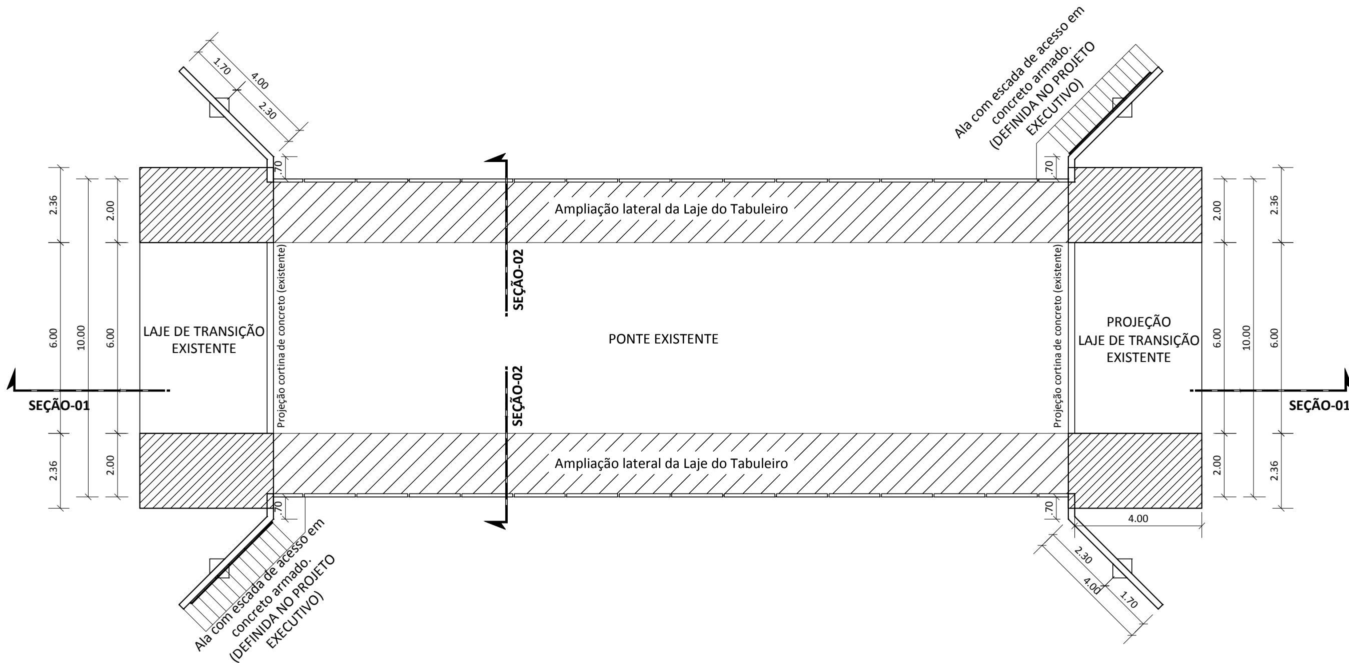
PLANTA BAIXA ESQUEMÁTICA DE AMPLIAÇÃO - PONTE IGARAPÉ IPÊPAQUI
