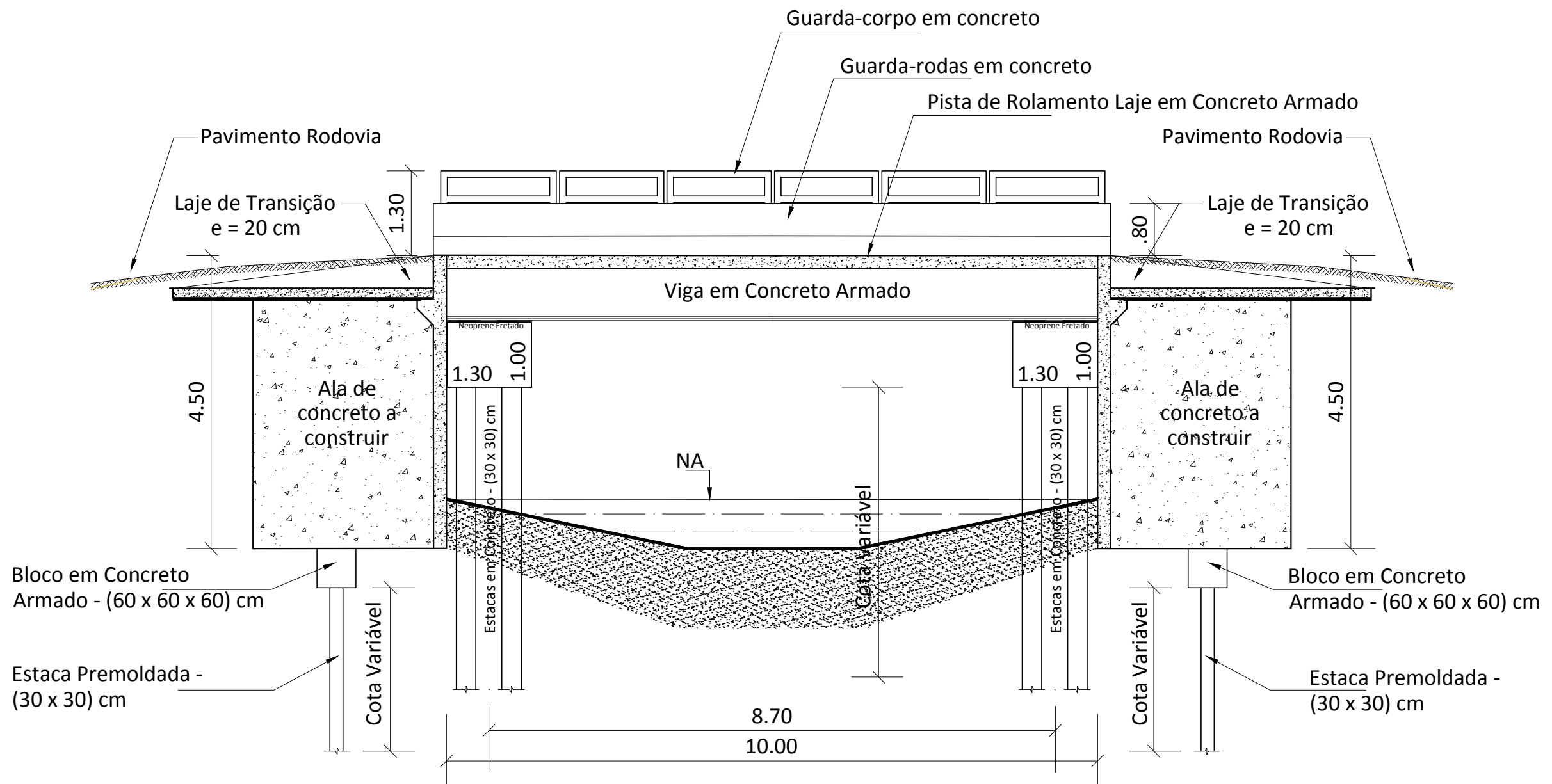
SEÇÃO 01 - LONGITUDINAL Escala: 1/75
