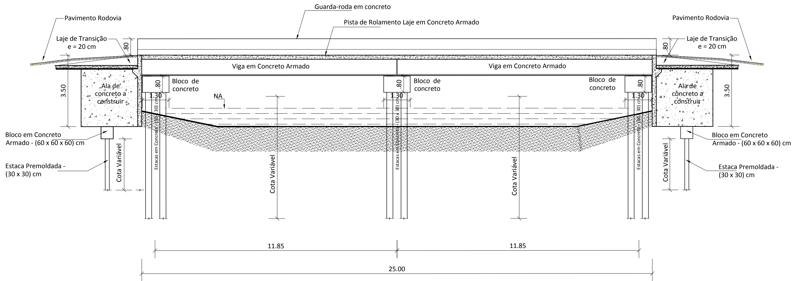
SEÇÃO 01 - LONGITUDINAL
