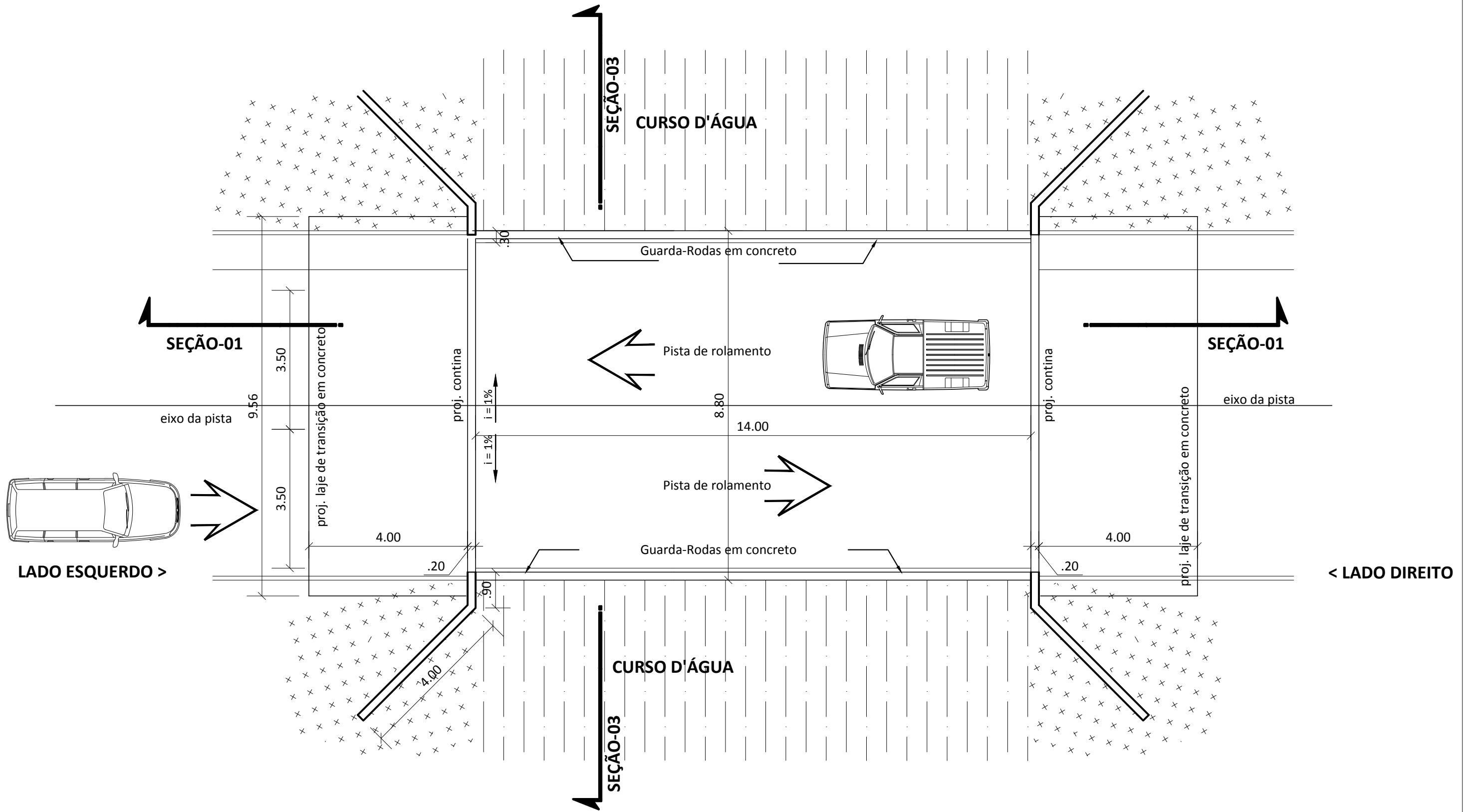
PLANTA ESQUEMÁTICA DA PONTE IGARAPÉ BUJARÚ ESC: 1/100
