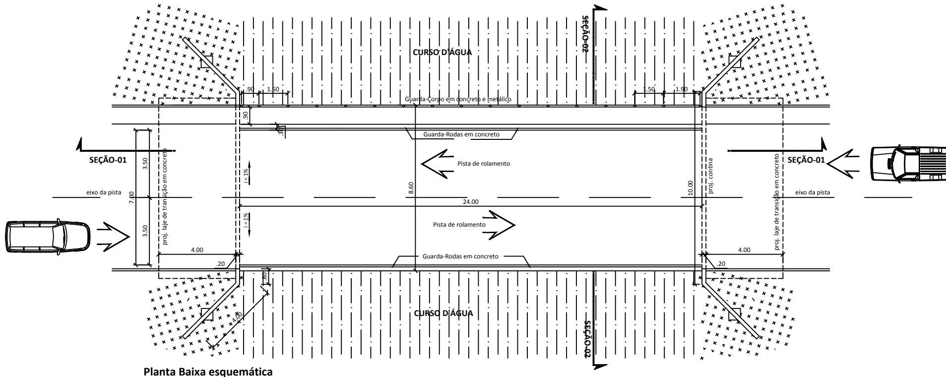
Planta Baixa esquemática
