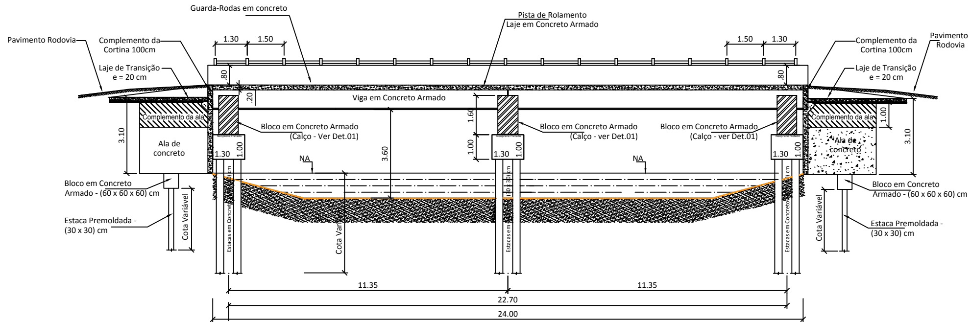
SEÇÃO 01 - LONGITUDINAL
