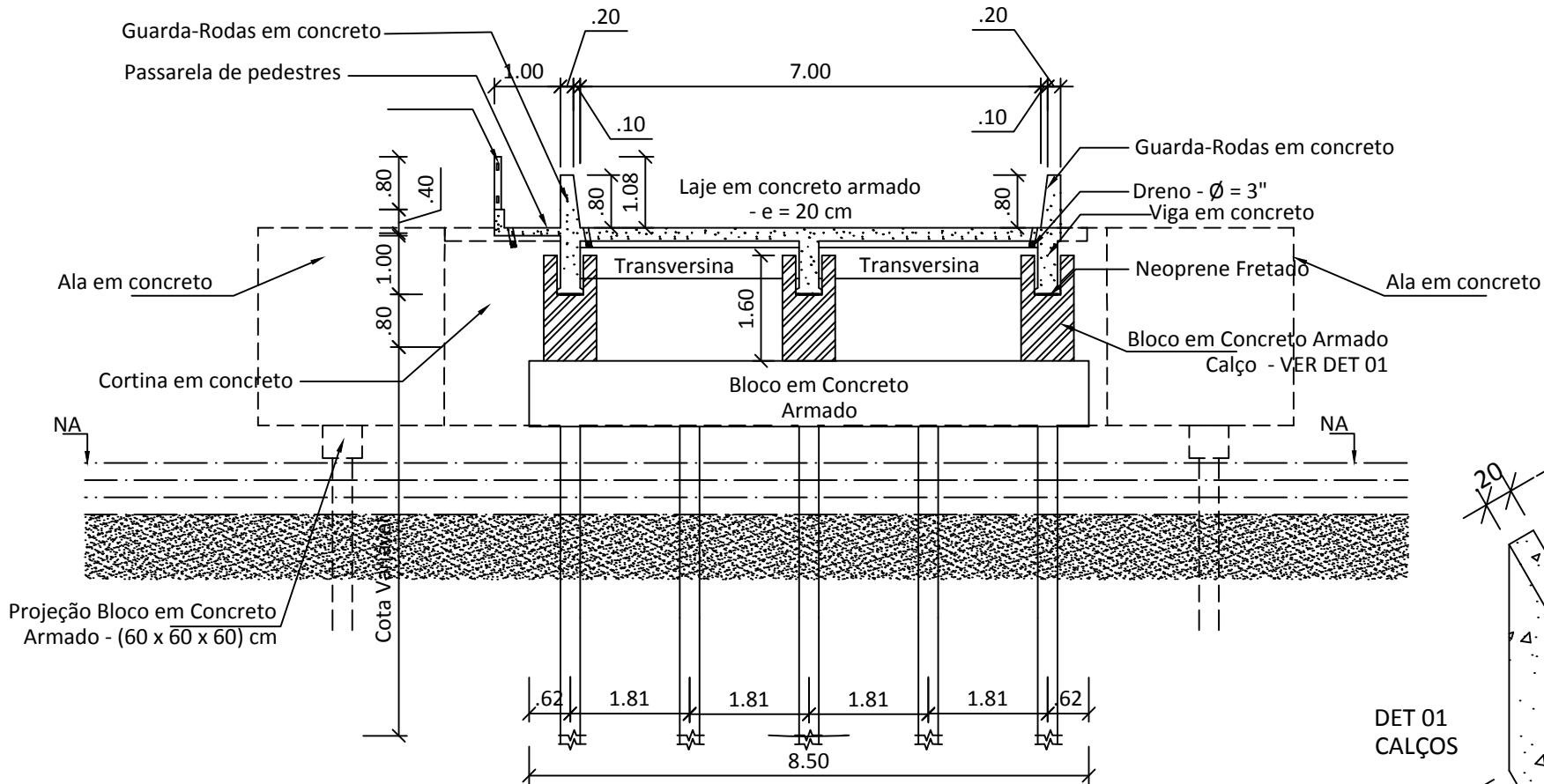
SEÇÃO 02 - TRANSVERSAL
