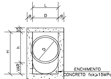
CORTE BB'
