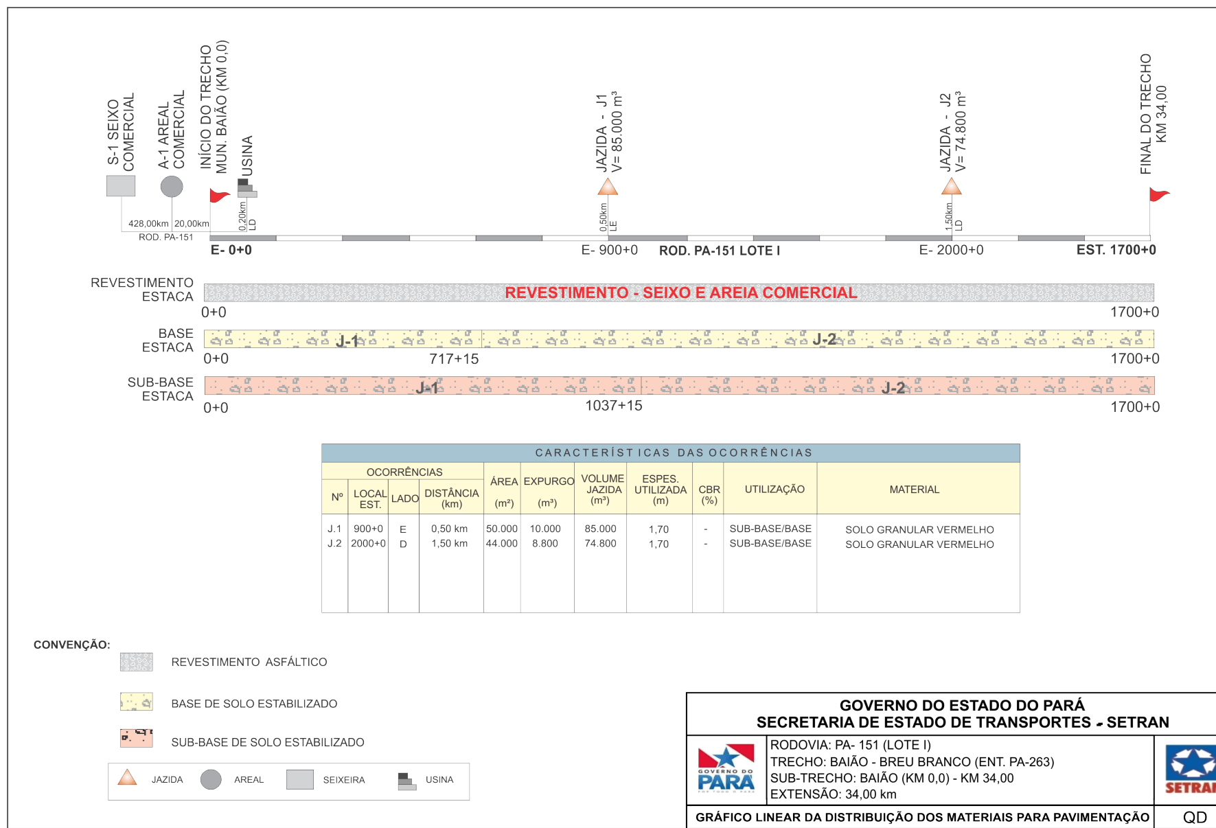
Figura 9 – Gráfico linear de distribuição dos materiais de pavimentação
