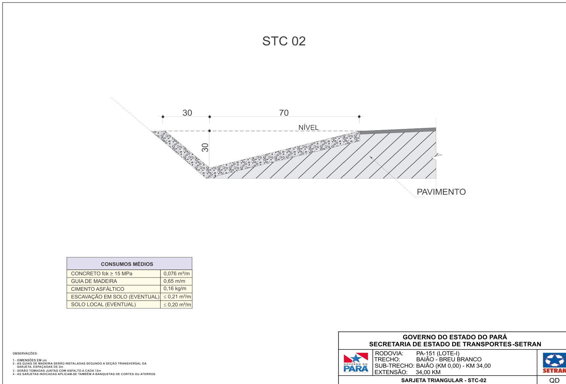
Figura 20 – Sarjeta Triangular de Concreto – STC-02
