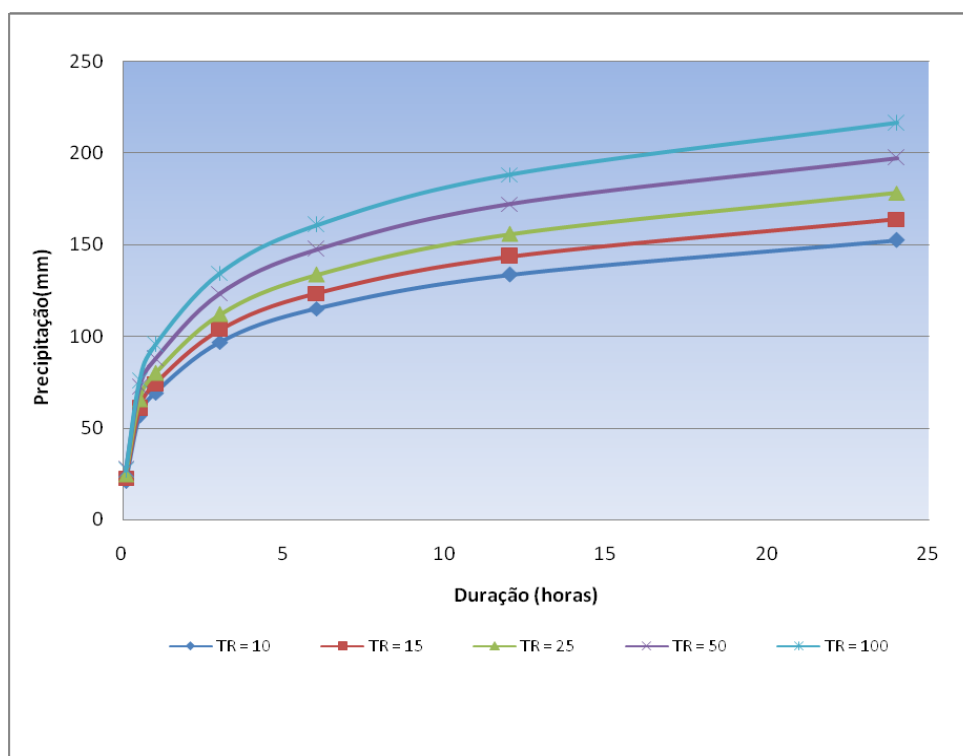
Figura 14 – Curvas Precipitação x Duração x Frequência
