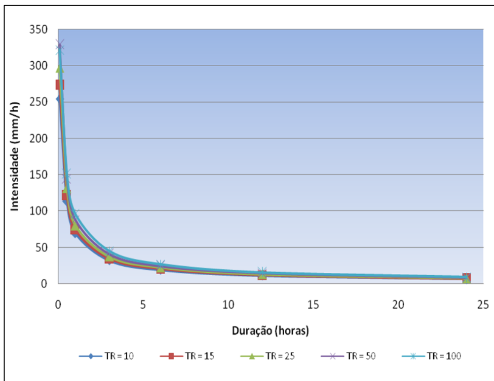
Figura 15 – Curvas Intensidade x Duração x Frequência
