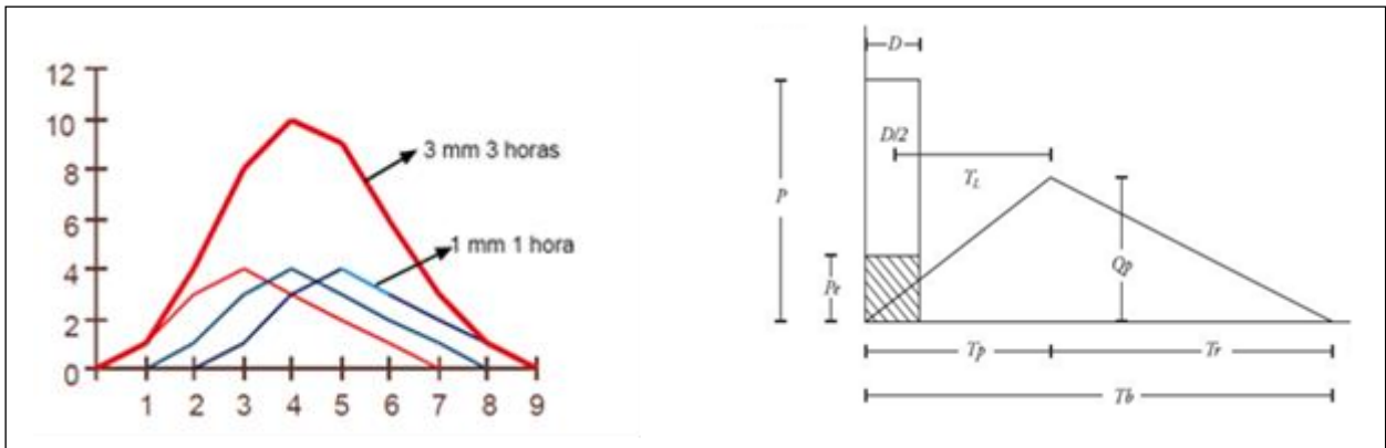
Figura 17 – Hidrograma Unitário Triangular
