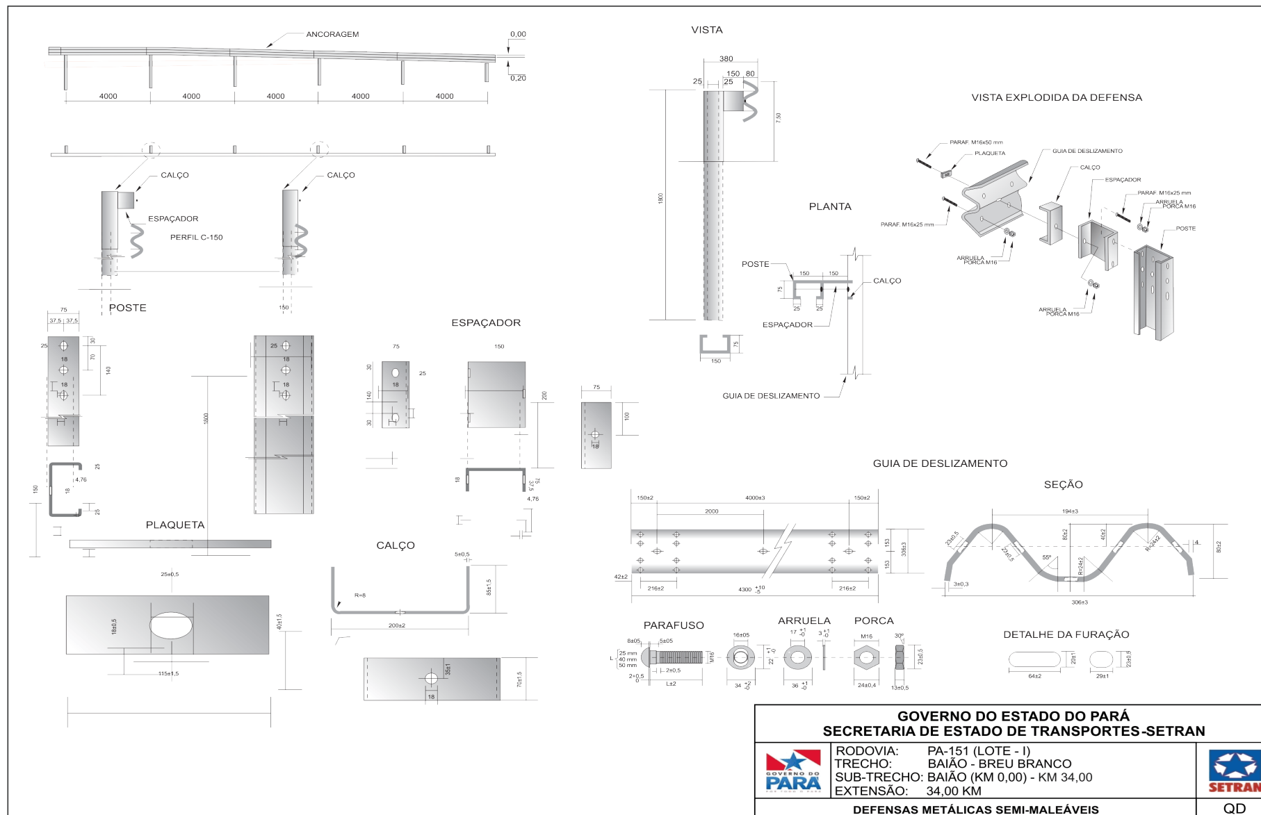
Figura 42 – Defensas Metálicas – Detalhamento
