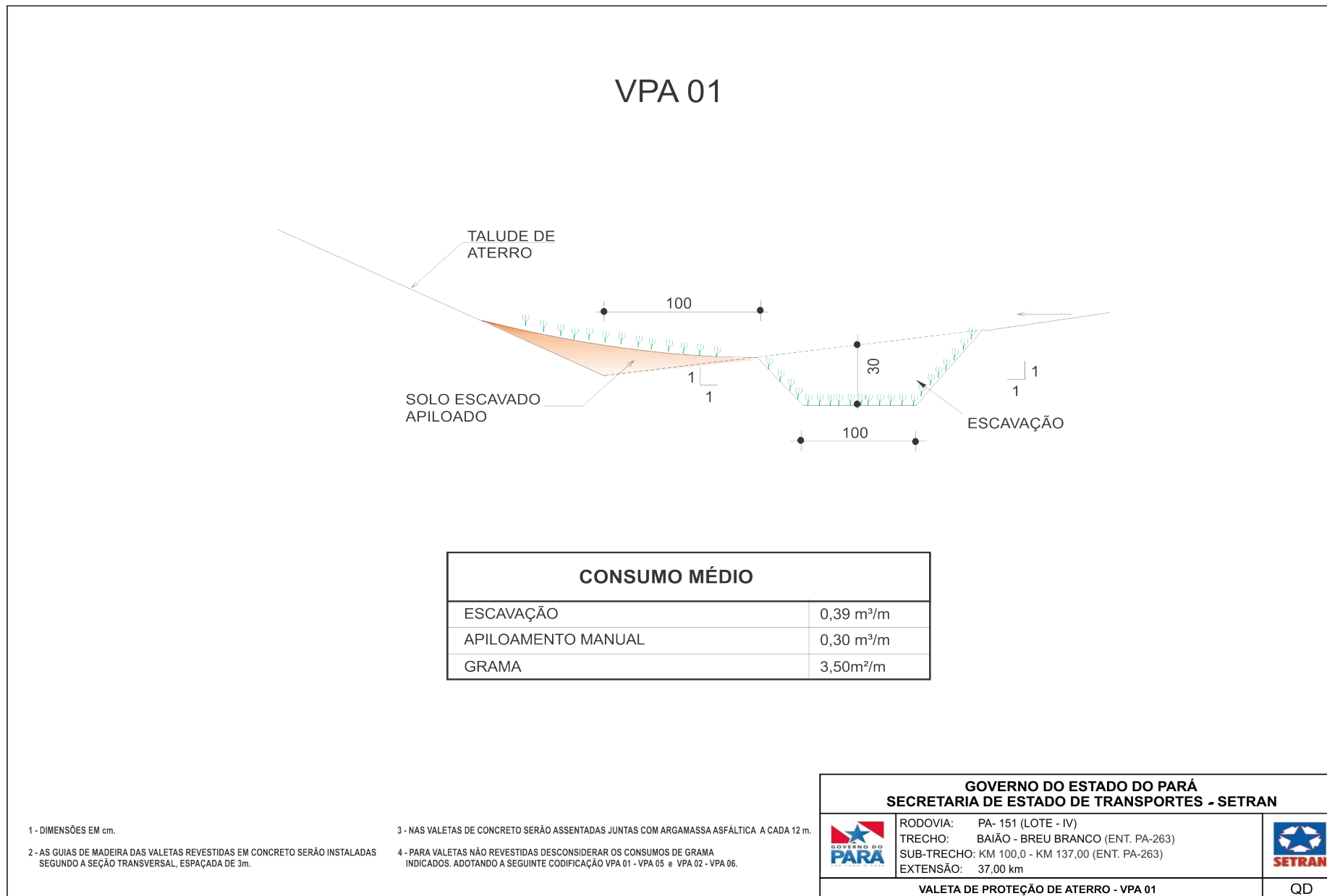
Figura 23 – Valeta de proteção de aterro – VPA-01
