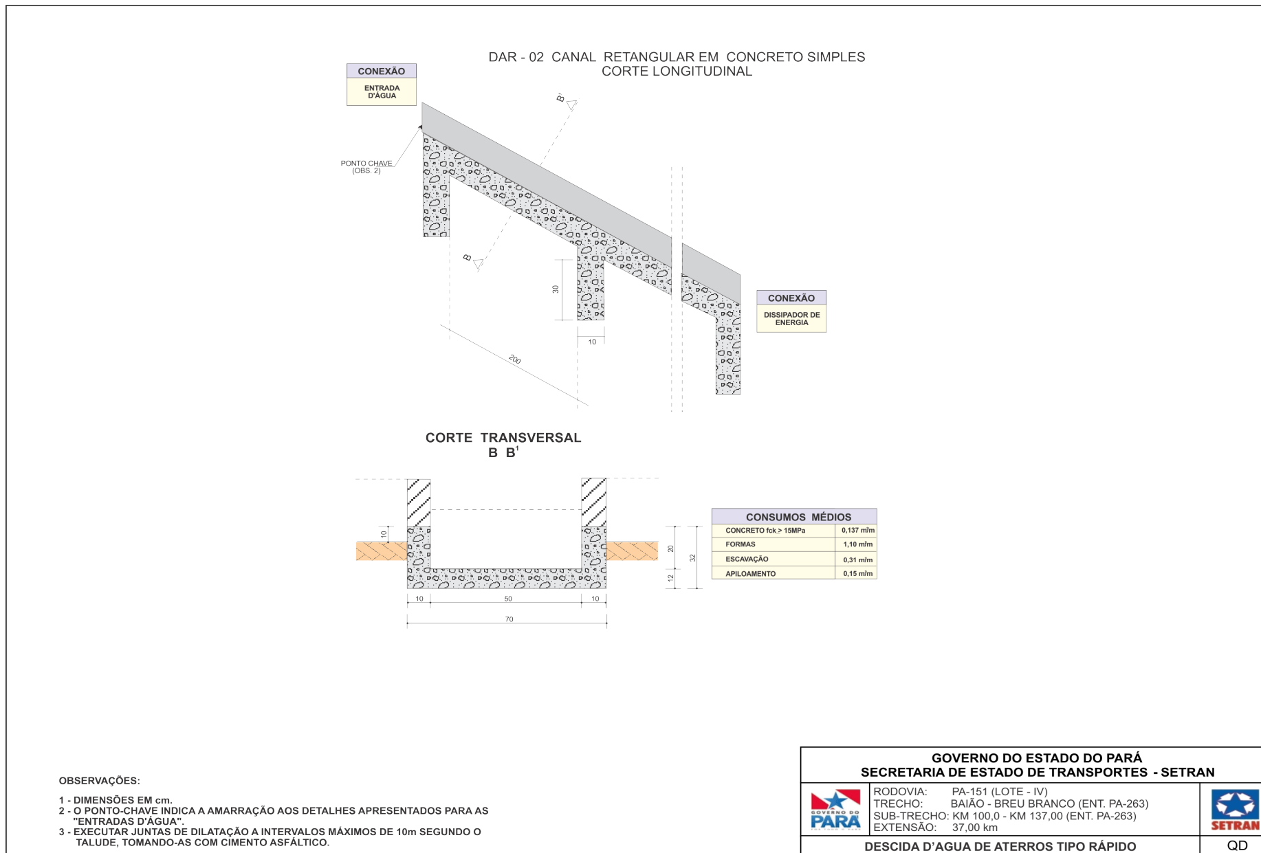
Figura 21 – Descida d’água de aterro tipo rápido
