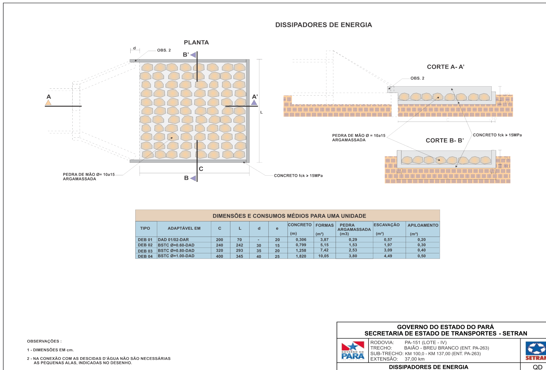
Figura 22 – Dissipadores de energia
