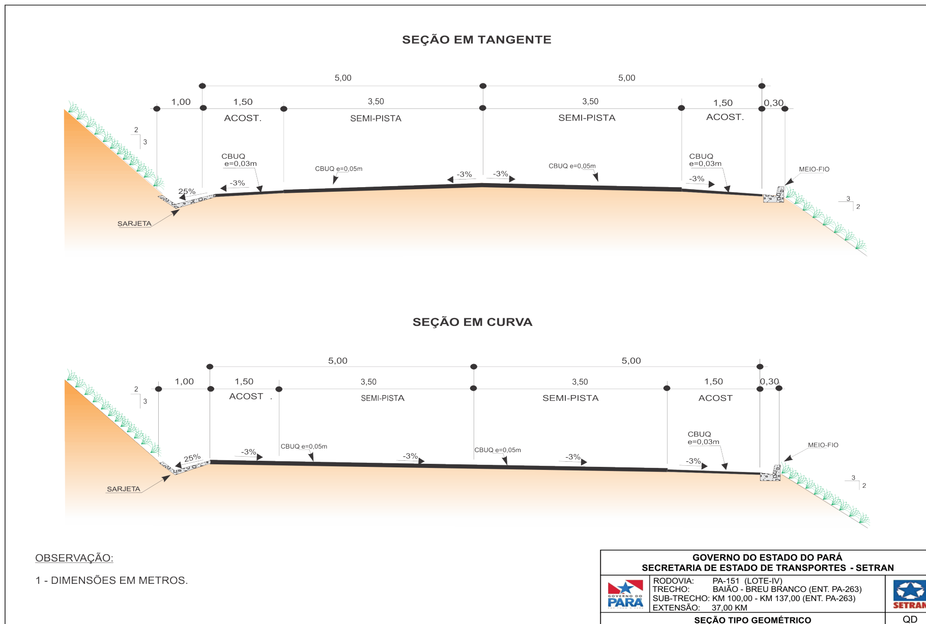
Figura 16 – Seção tipo do projeto geométrico
