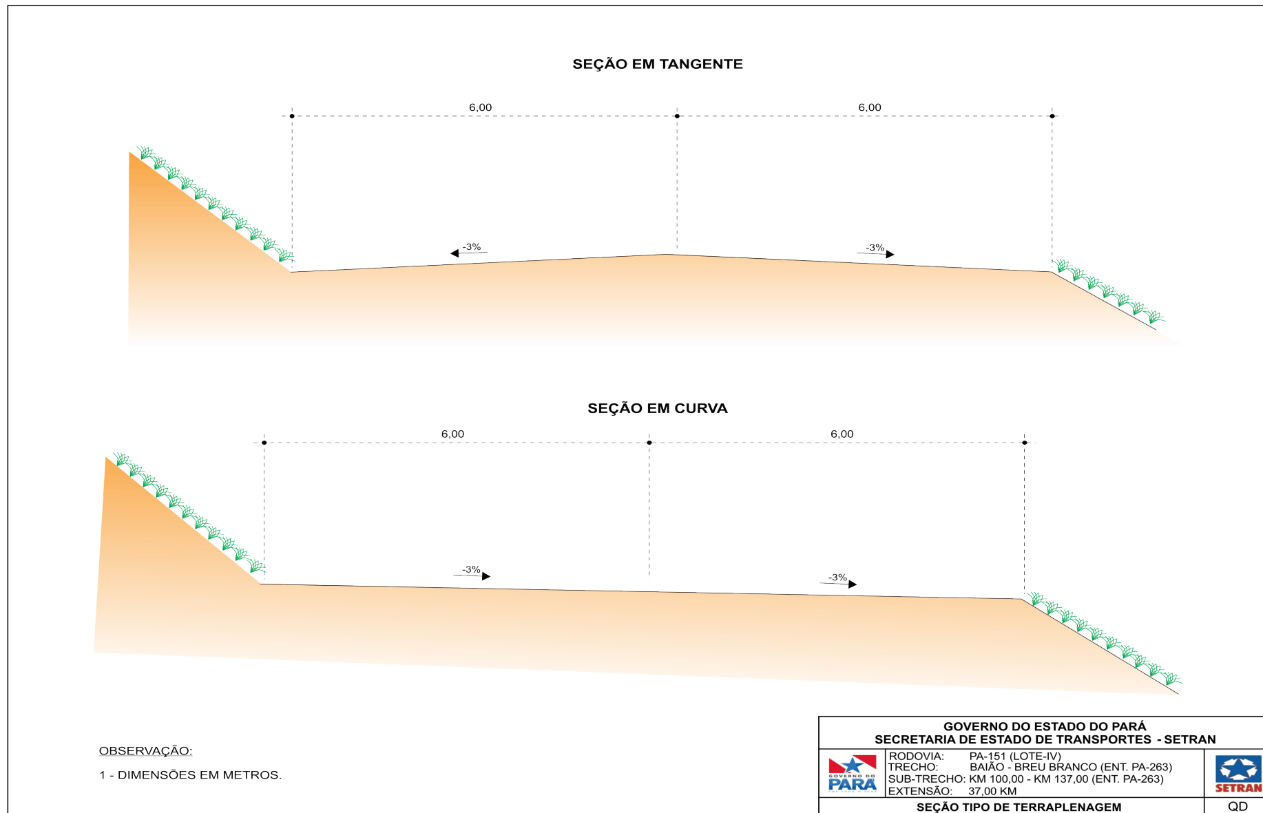
Figura 17 – Seção tipo do projeto de Terraplenagem
