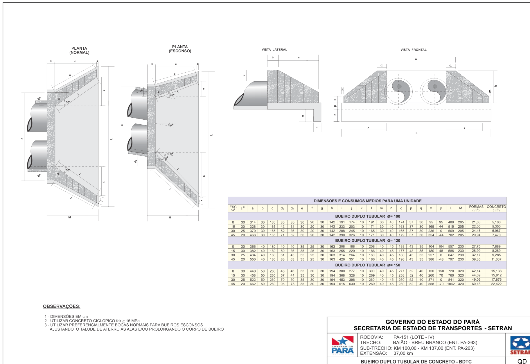
Figura 29 – BDTc bocas normais e esconsas
