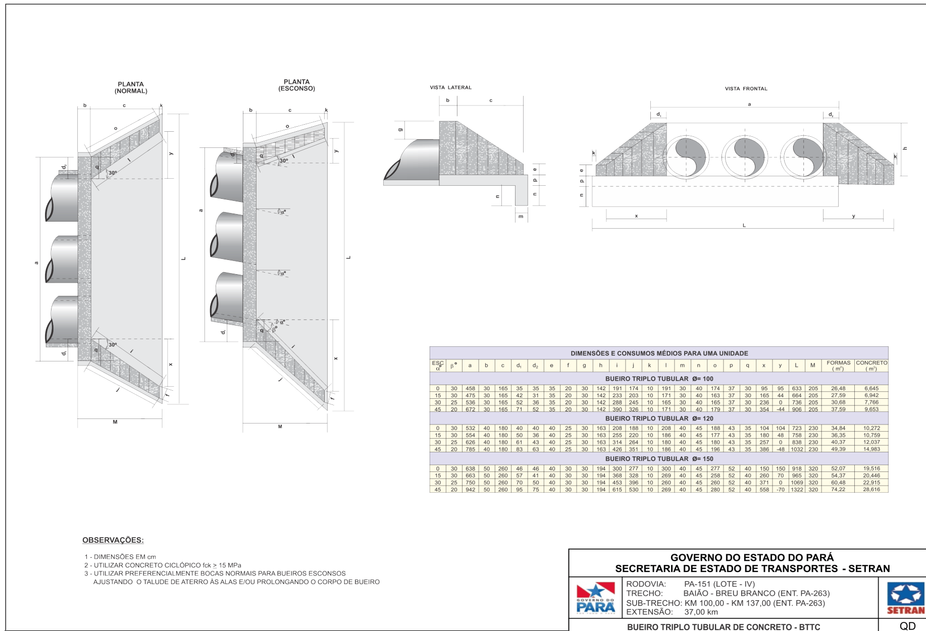
Figura 30 – BTTC bocas normais e esconsas
