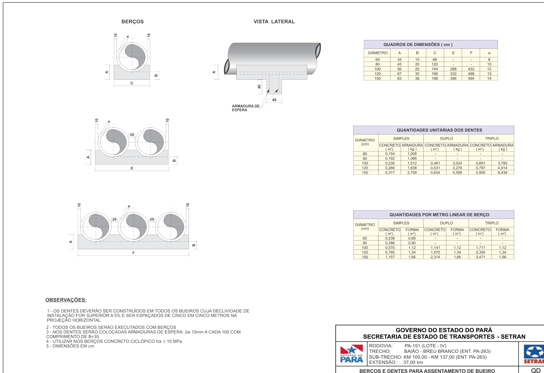
Figura 27 – Berços e dentes para assentamento de bueiros
