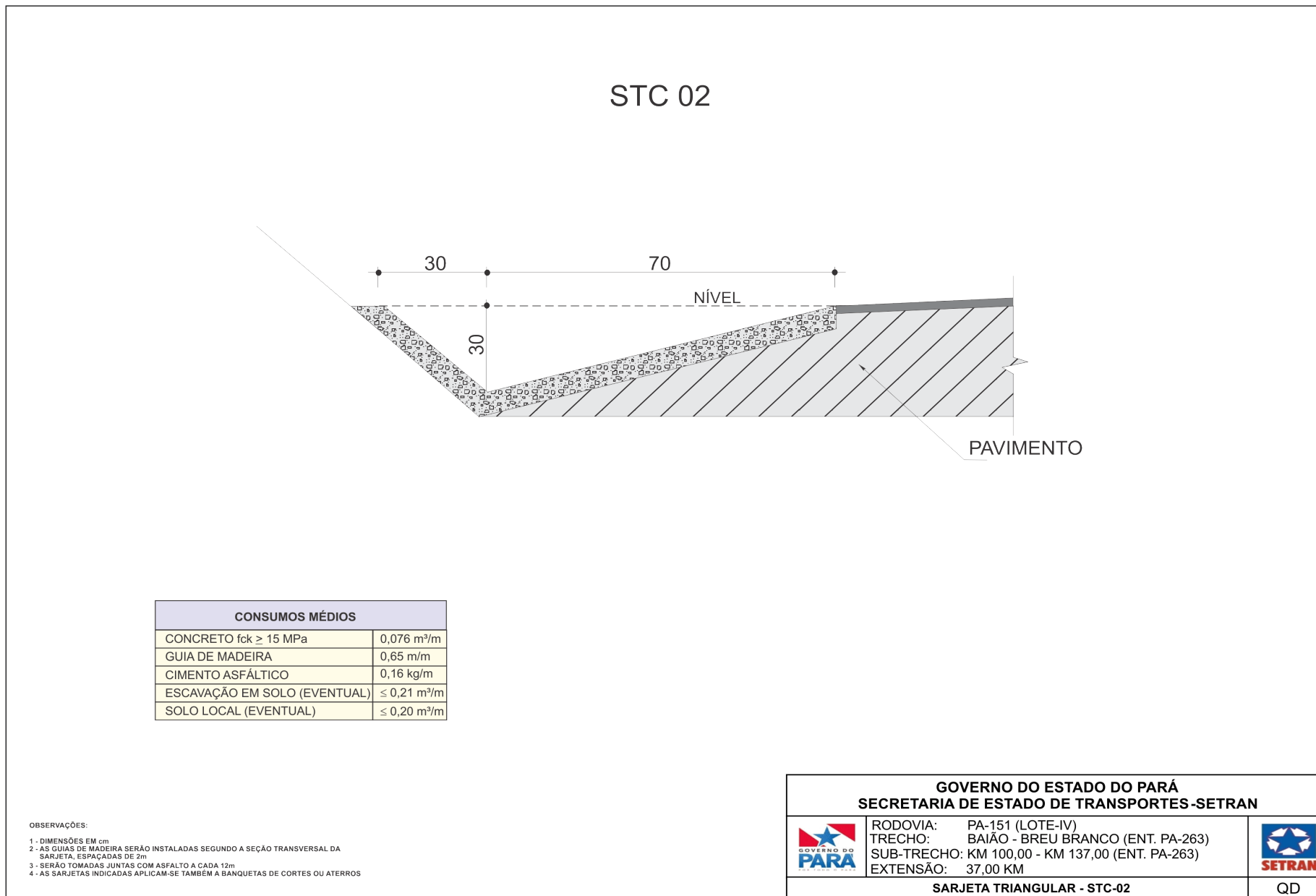
Figura 18 – Sarjeta Triangular de Concreto – STC-02
