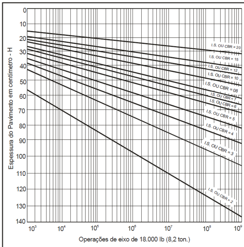
Figura 31 – Ábaco de Dimensionamento do DNIT, 2006.
