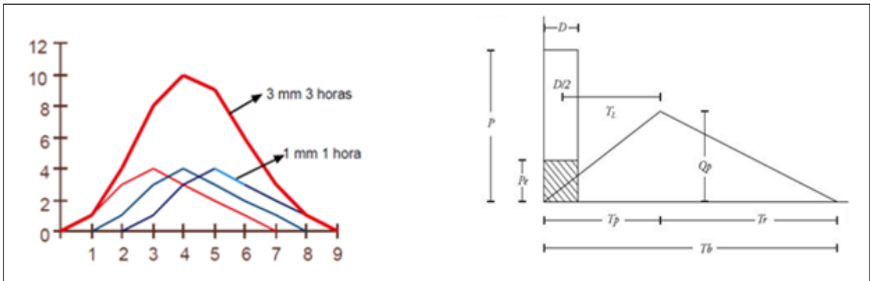
Figura 15 – Hidrograma Unitário Triangular
