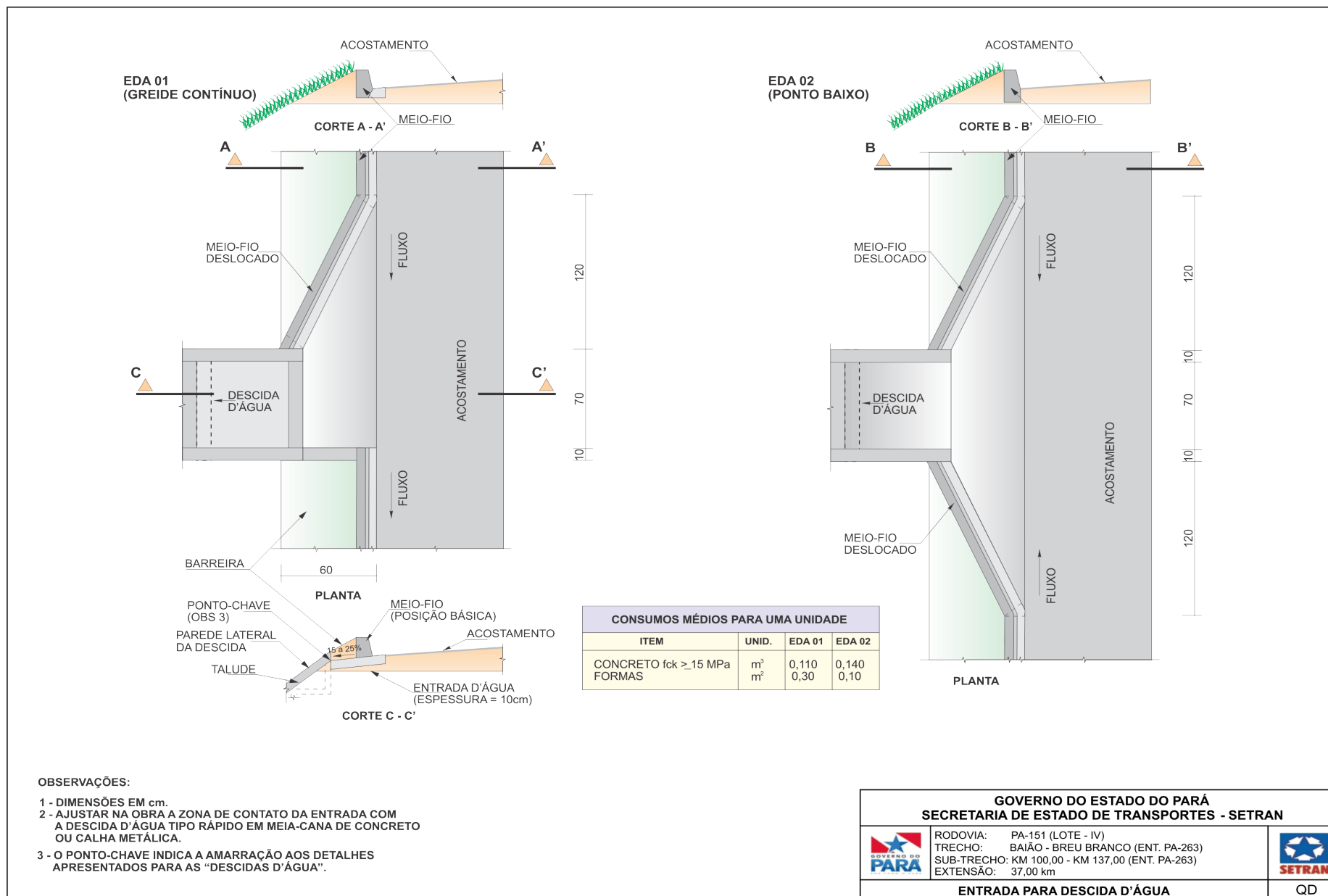
Figura 20 – Entrada para descida d'água
