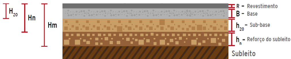
Figura 32 – Simbologia das camadas do pavimento DNIT, 2006.
