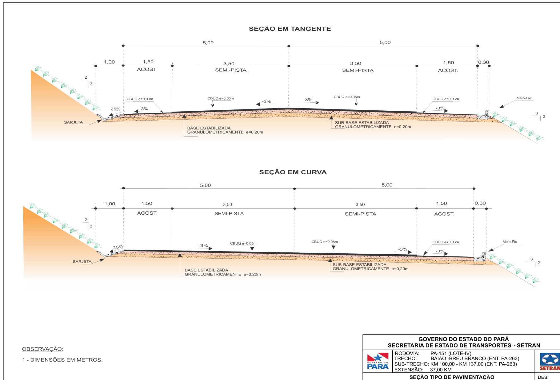
Figura 35 – Seção tipo de Pavimentação
