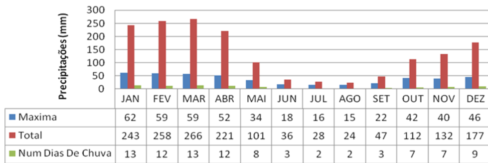
Figura 10 – Histograma das precipitações médias no período de 1984 a 2004
