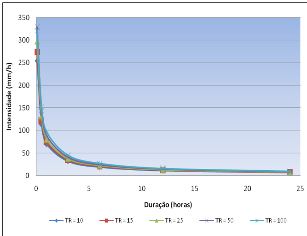
Figura 13 – Curvas Intensidade x Duração x Frequência
