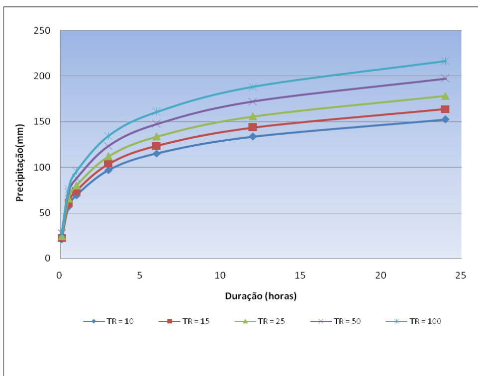
Figura 12 – Curvas Precipitação x Duração x Frequência
