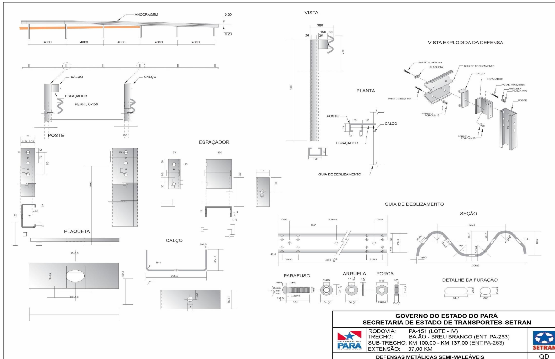
Figura 40 – Defensas Metálicas – Detalhamento
