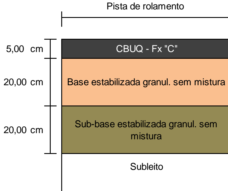
Figura 34 – Linear da Pista de rolamento
