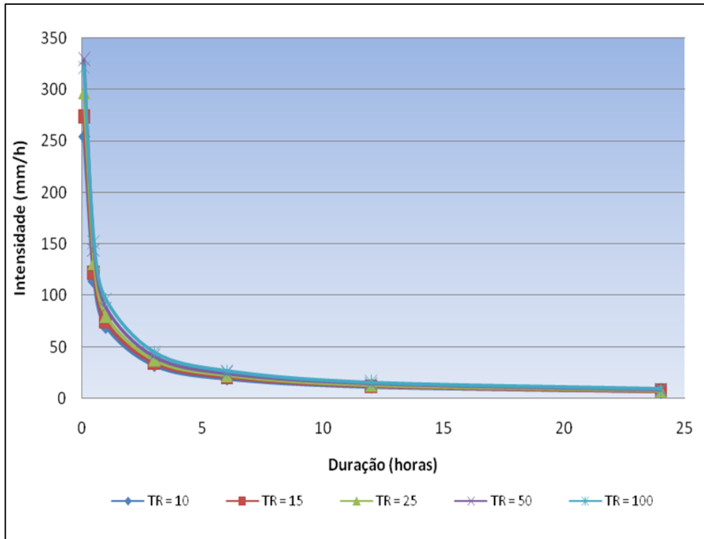
Figura 15 – Curvas Intensidade x Duração x Frequência
