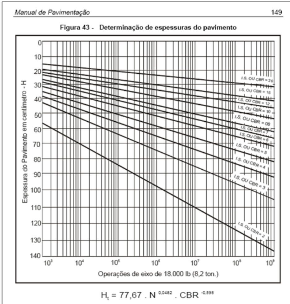
Figura 33 – Ábaco determinação de espessuras do pavimento
