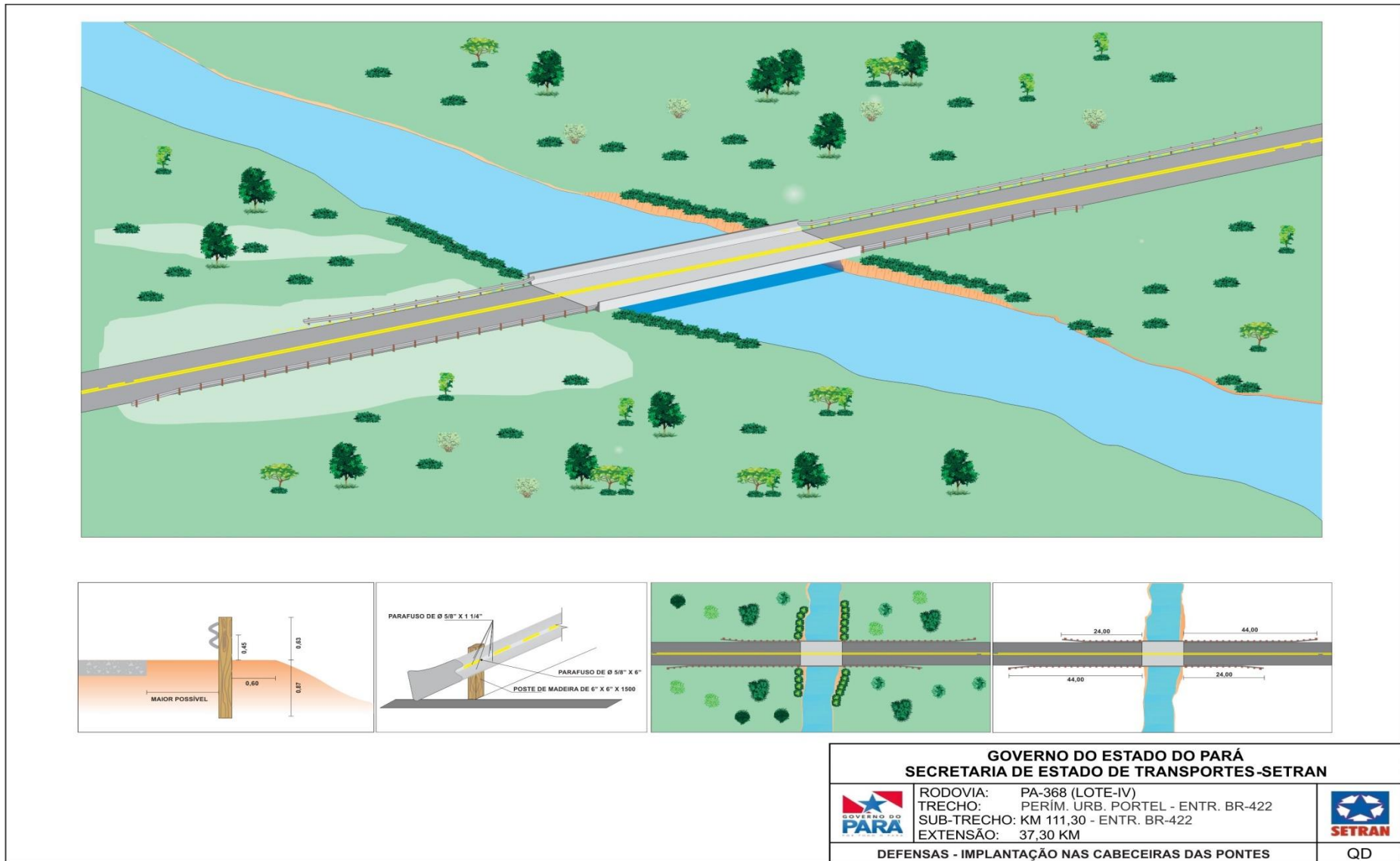
Figura 40 – Defensas metálicas – Implantação
