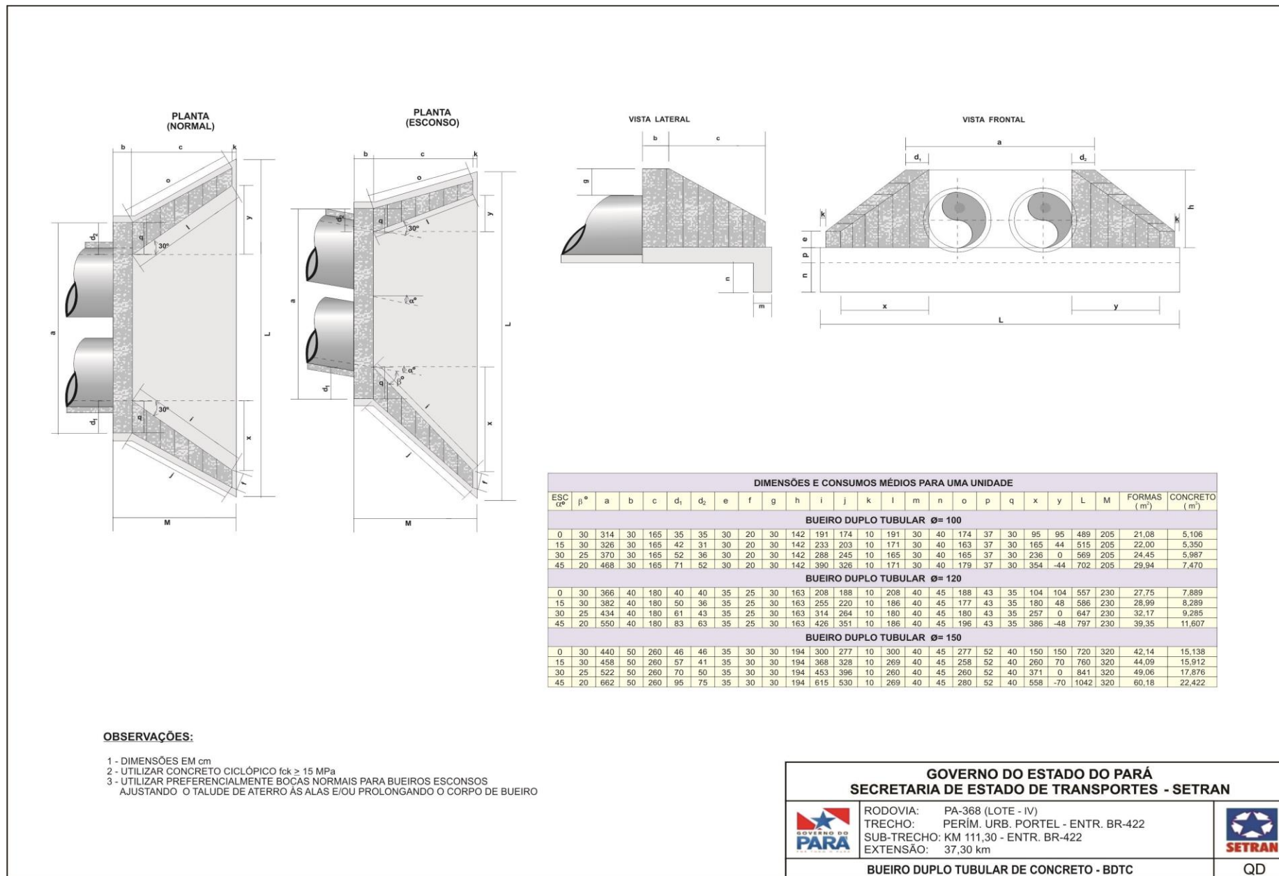
Figura 31 – BDC bocas normais e esconso
