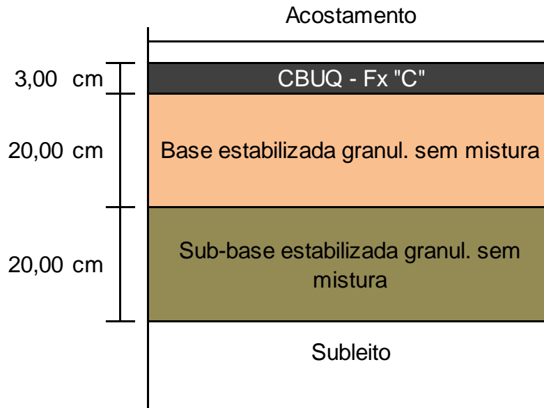
Figura 35 – Linear de Acostamento
