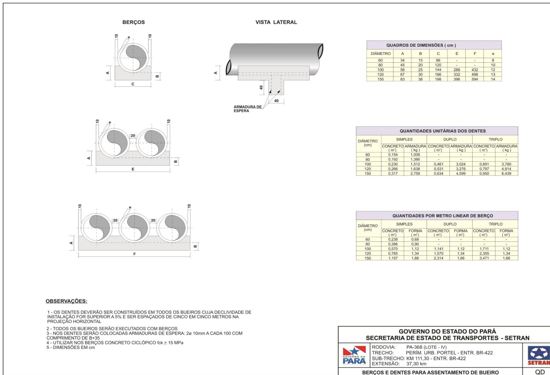
Figura 29 – Berços e dentes para assentamento de bueiros
