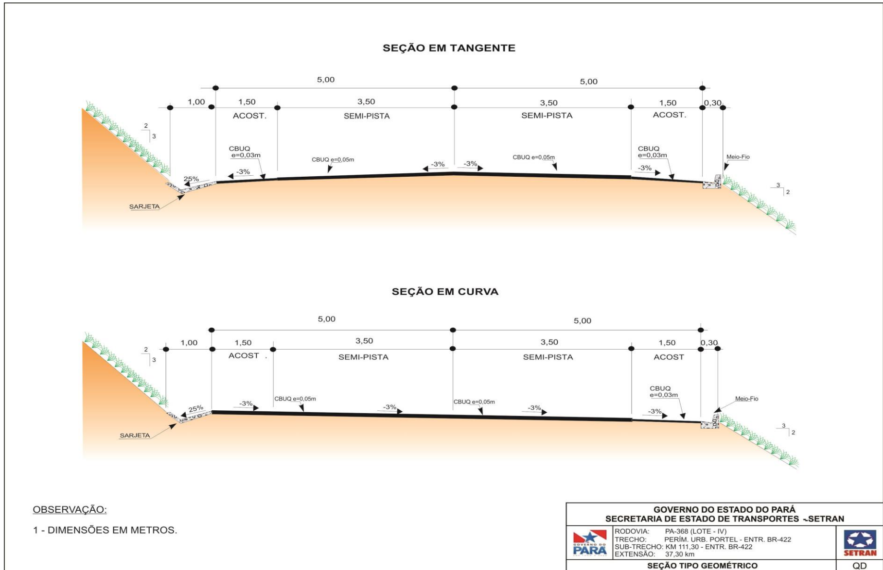
Figura 18 – Seção tipo do projeto geométrico
