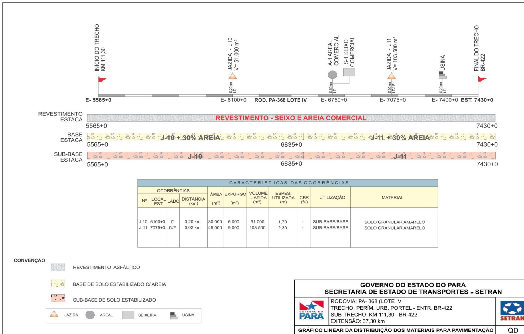
Figura 9 – Gráfico linear de distribuição dos materiais de pavimentação
