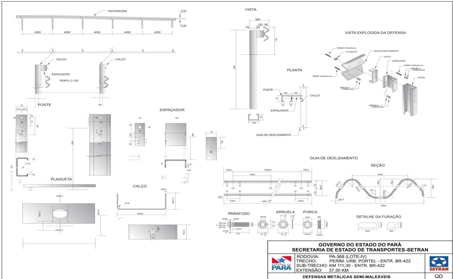
Figura 41 – Defensas metálicas – Detalhamento
