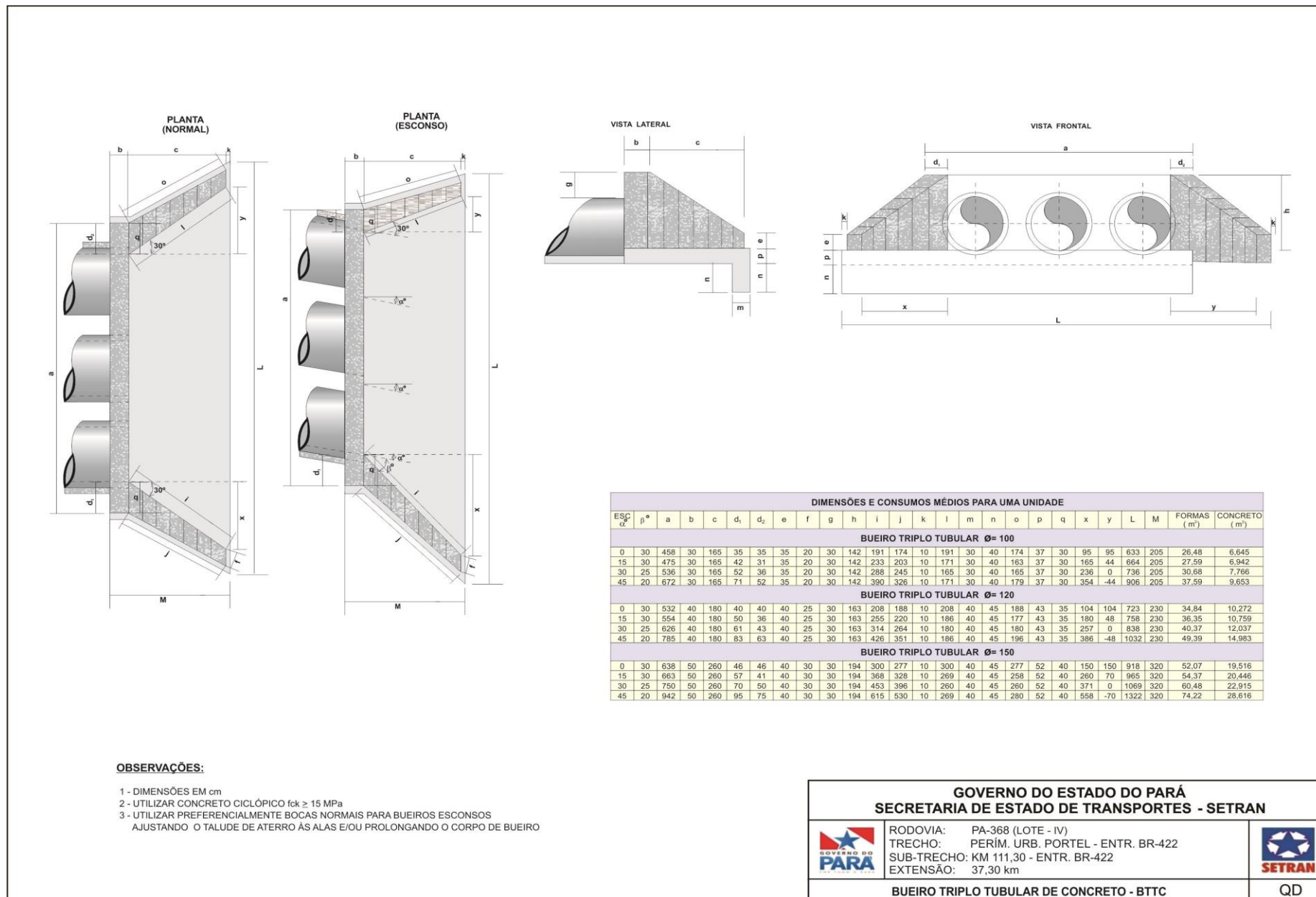
Figura 32 – BTTC bocas normais e esconso
