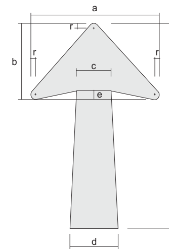
SETA VERTICAL OU DIAGONAL PARA DUAS LINHAS
