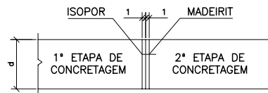
DETALHE DA JUNTA DE DILATAÇÃO
