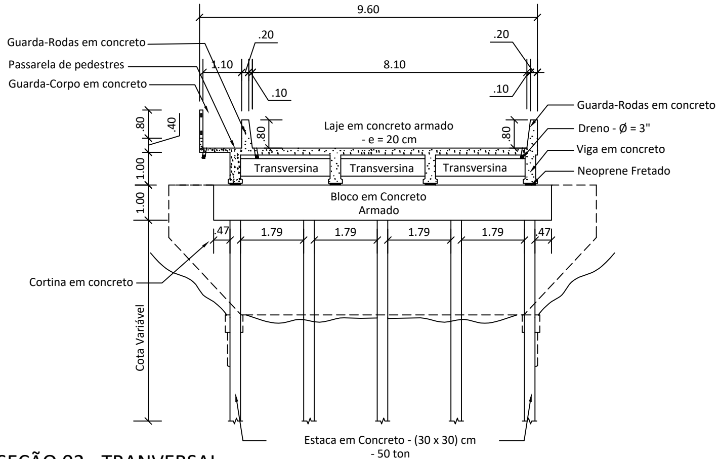
SEÇÃO 02 - TRANVERSAL
