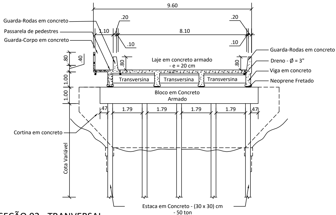
SEÇÃO 02 - TRANVERSAL
