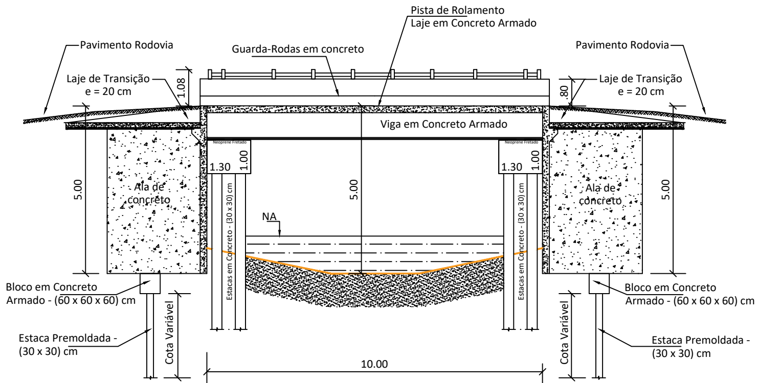
SEÇÃO 01 - LONGITUDINAL
