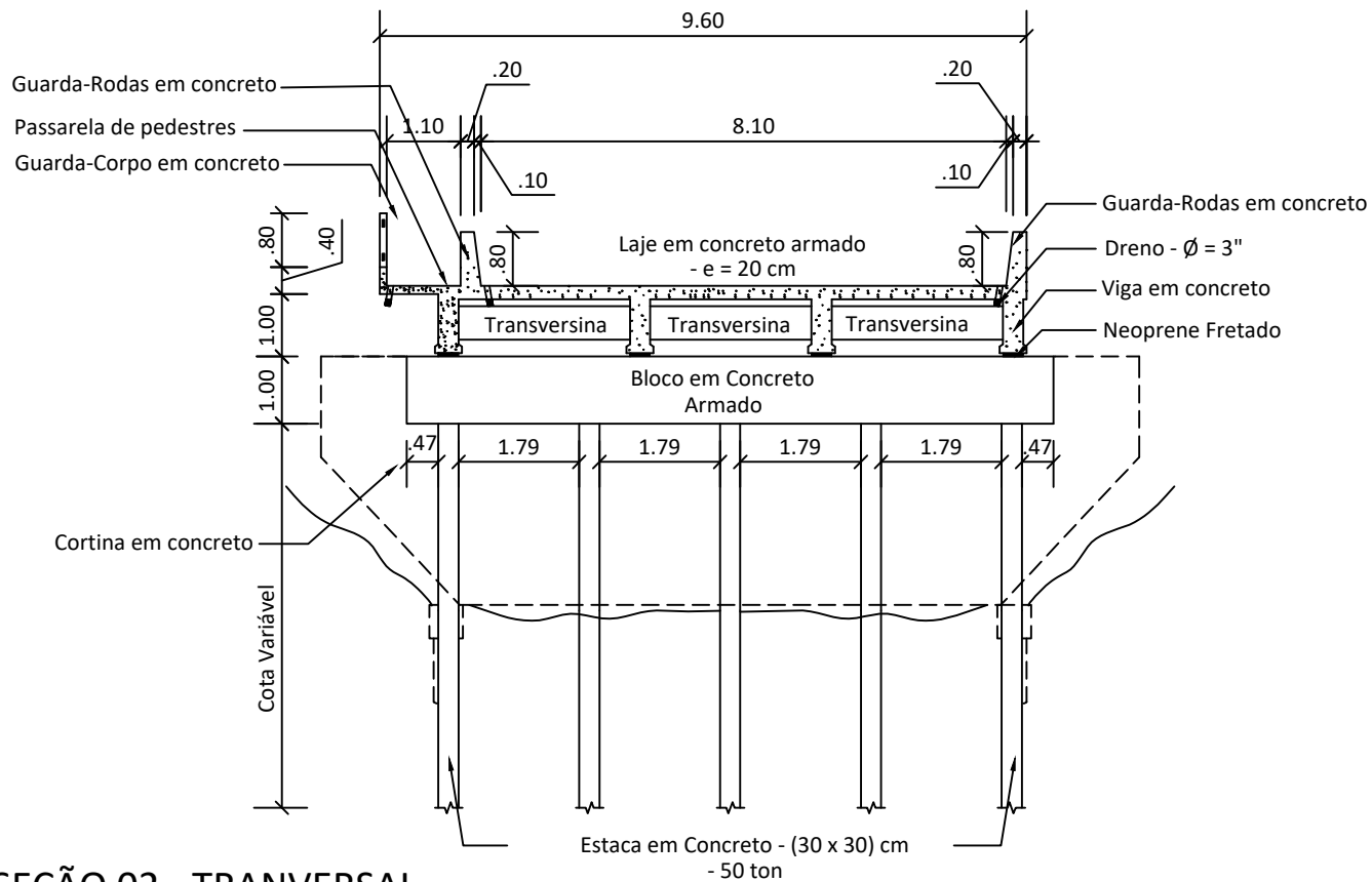
SEÇÃO 02 - TRANVERSAL
