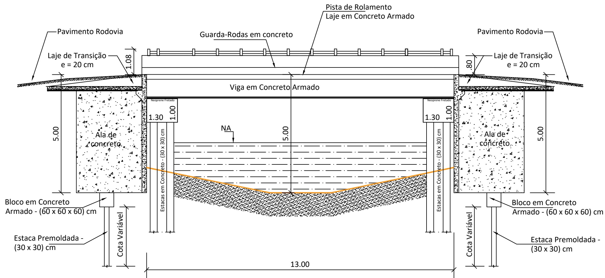
SEÇÃO 01 - LONGITUDINAL
