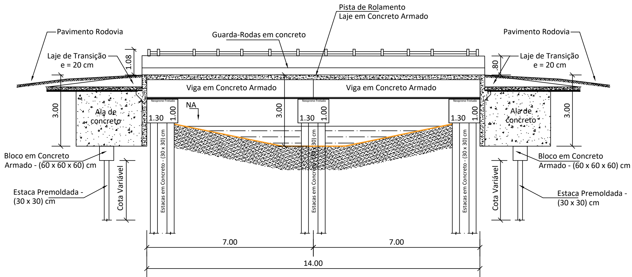
SEÇÃO 01 - LONGITUDINAL
