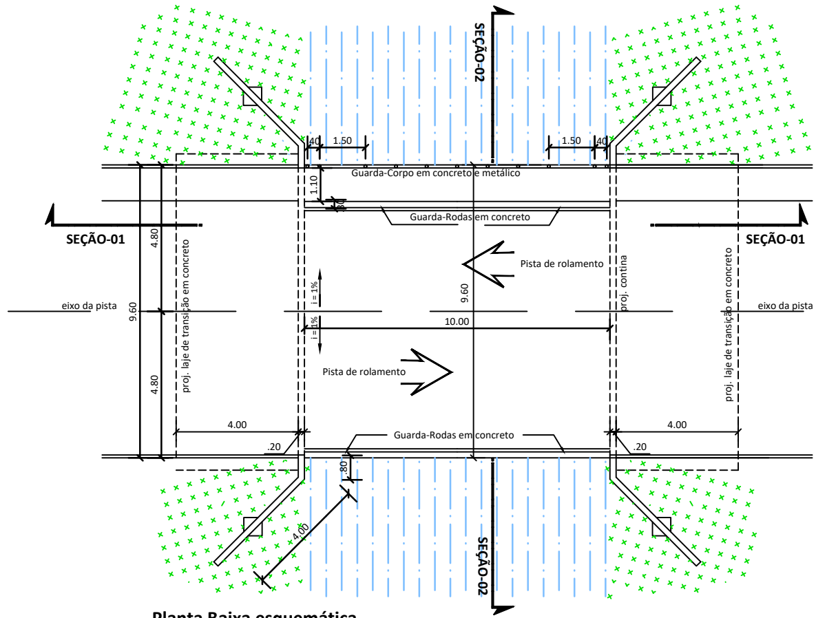
Planta Baixa esquemática
