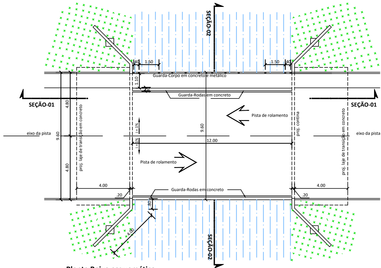
Planta Baixa esquemática
