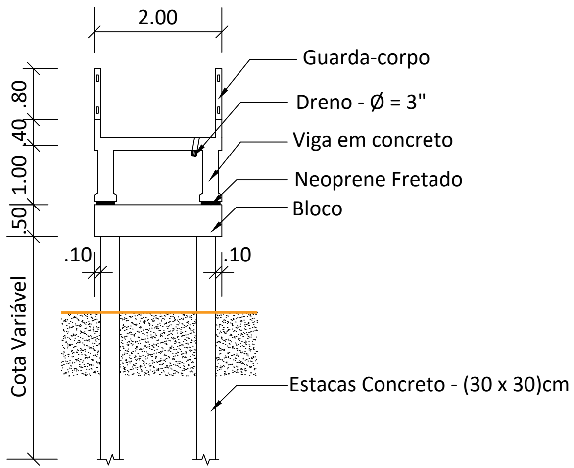
SEÇÃO 02 - TRANVERSAL
