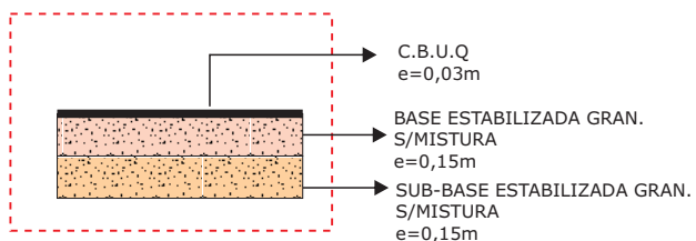
ESTRUTURA DO PAVIMENTO - SEMI-PISTA / FX. DE SEG.
