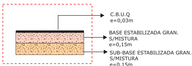
ESTRUTURA DO PAVIMENTO - ACOSTAMENTO / CICLOVIA
