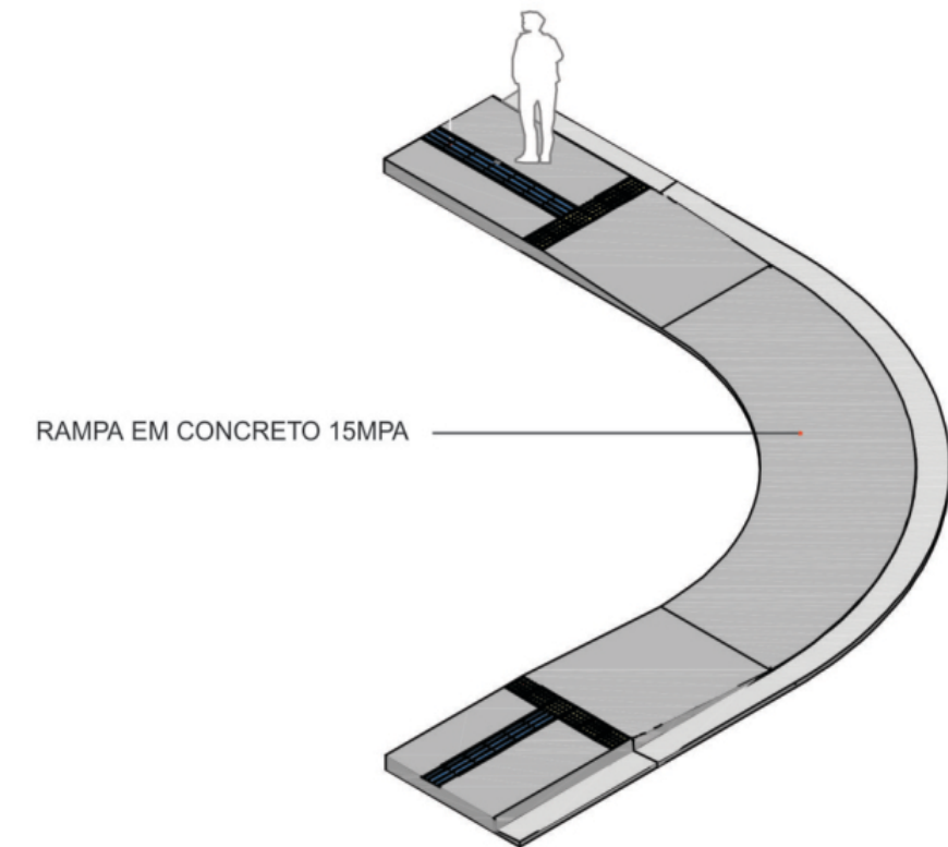
5 DIAGRAMA CALÇADA CURVA Esc 1:75
