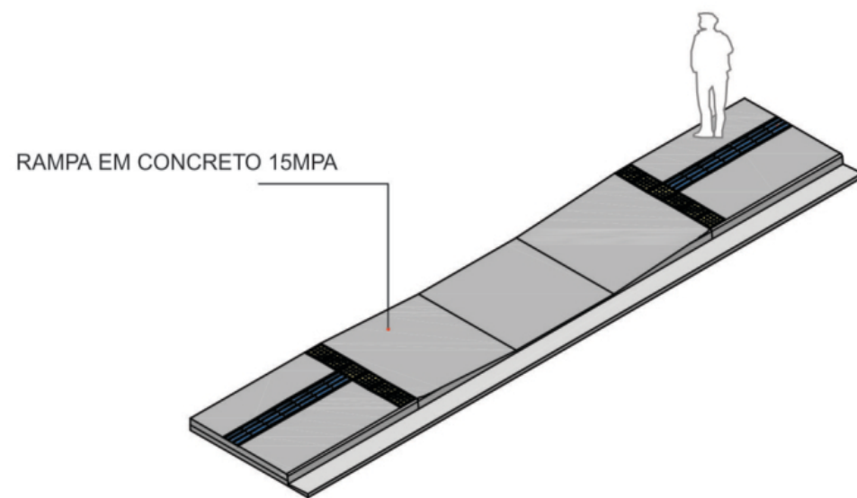
3 DIAGRAMA CALÇADA RETA Esc 1:75
