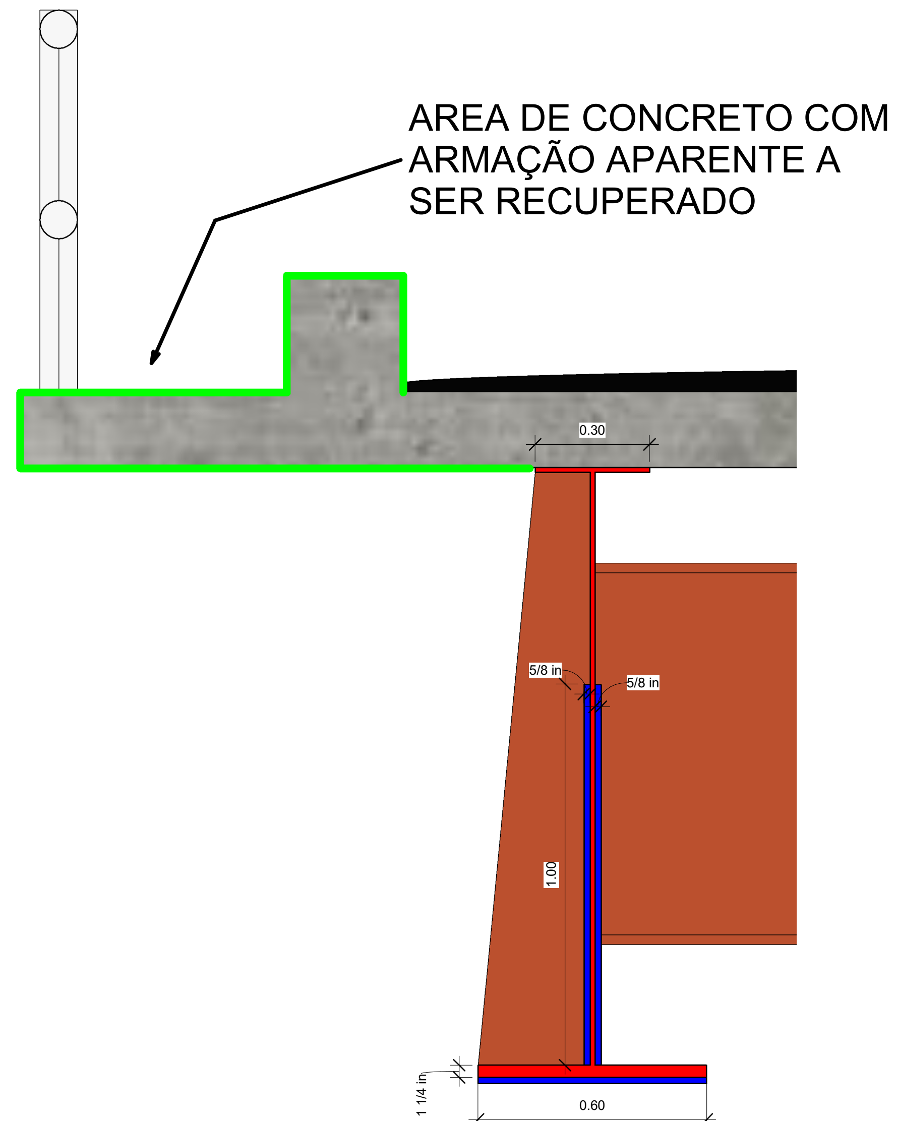
3 DETALHE DO REFORÇO 1 : 10
