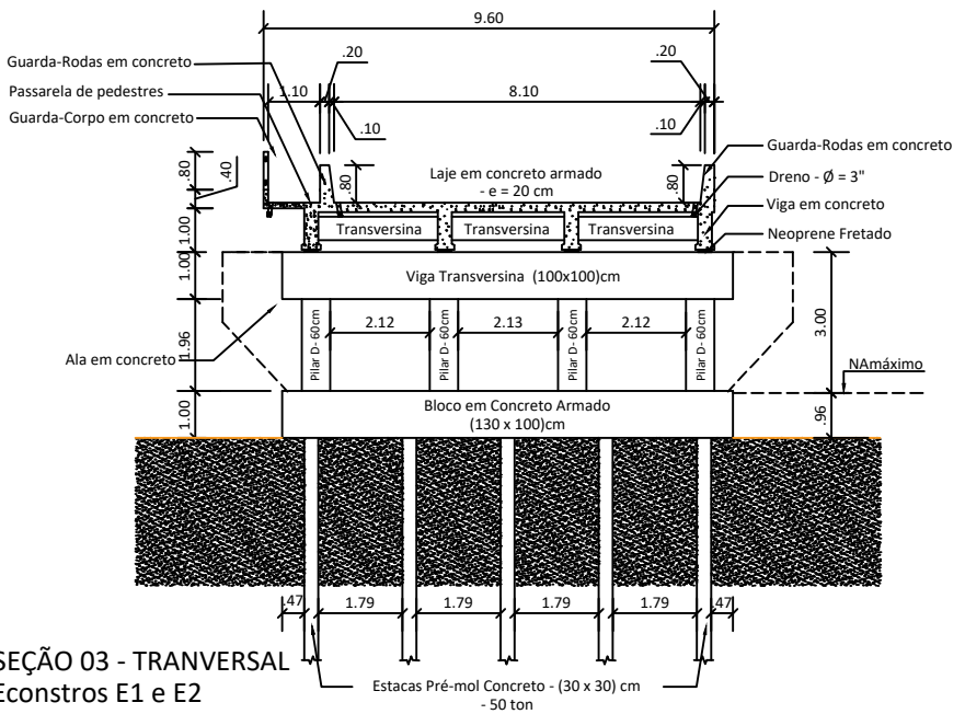
SEÇÃO 02 - TRANVERSAL Trechos corrente
