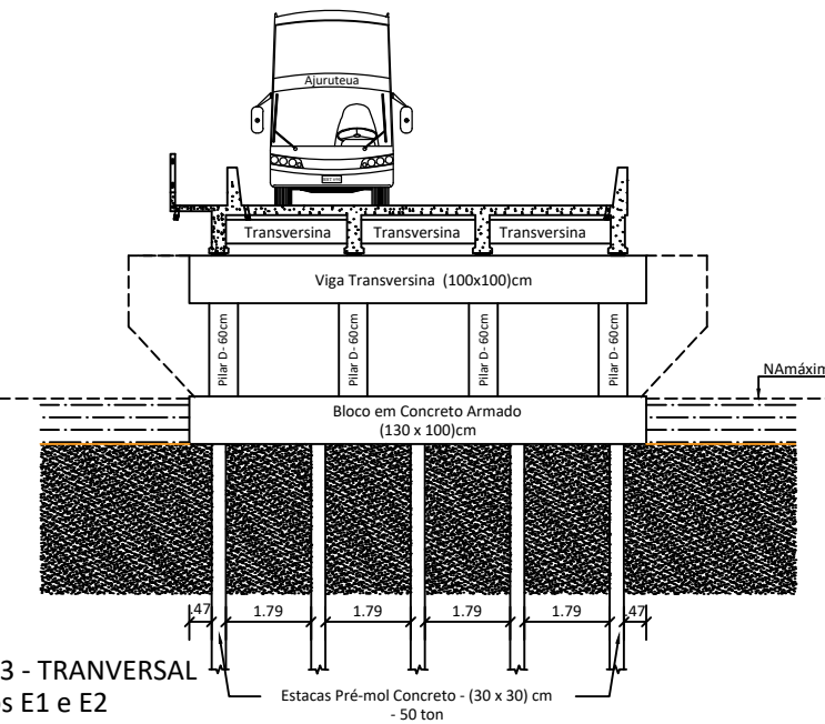
SEÇÃO 02 - TRANVERSAL TRECHO CORRENTE
